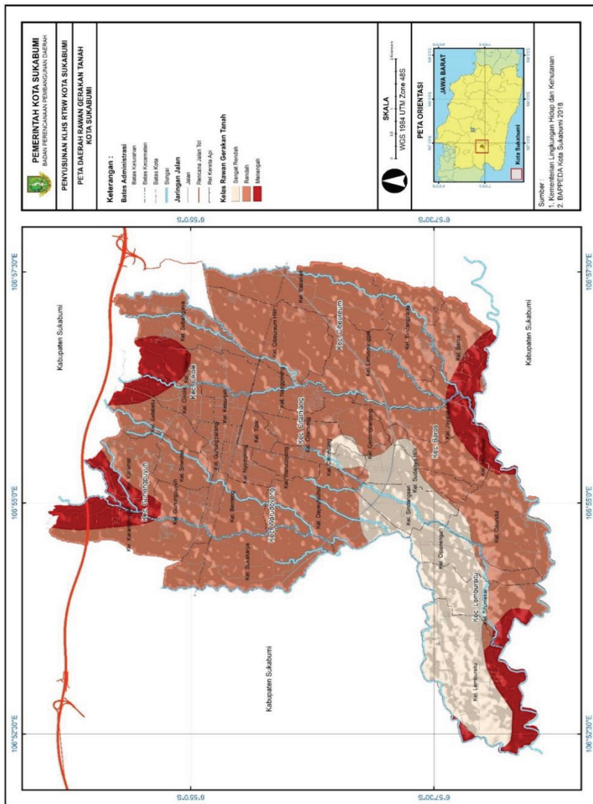
Gambar 2.6 Peta Rawan Gerakan Tanah di Daerah
