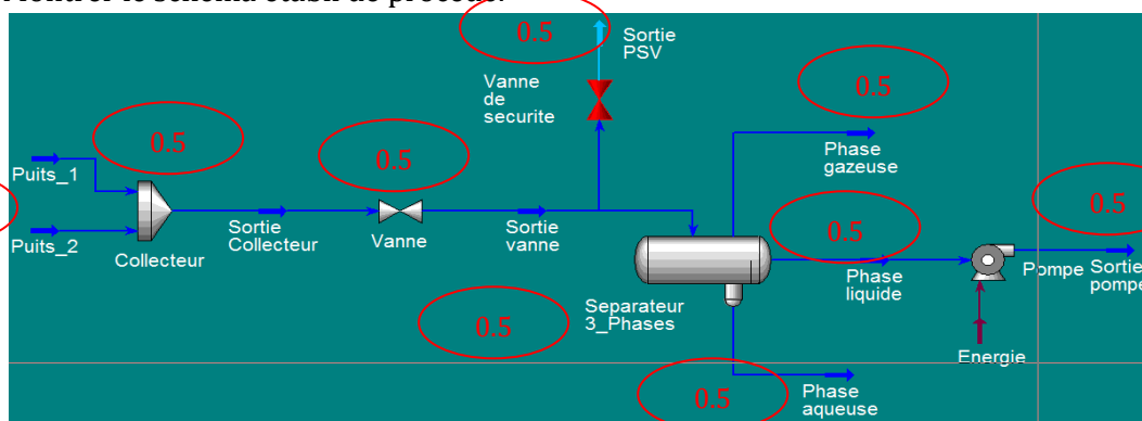
Schéma de fluide de procédé
