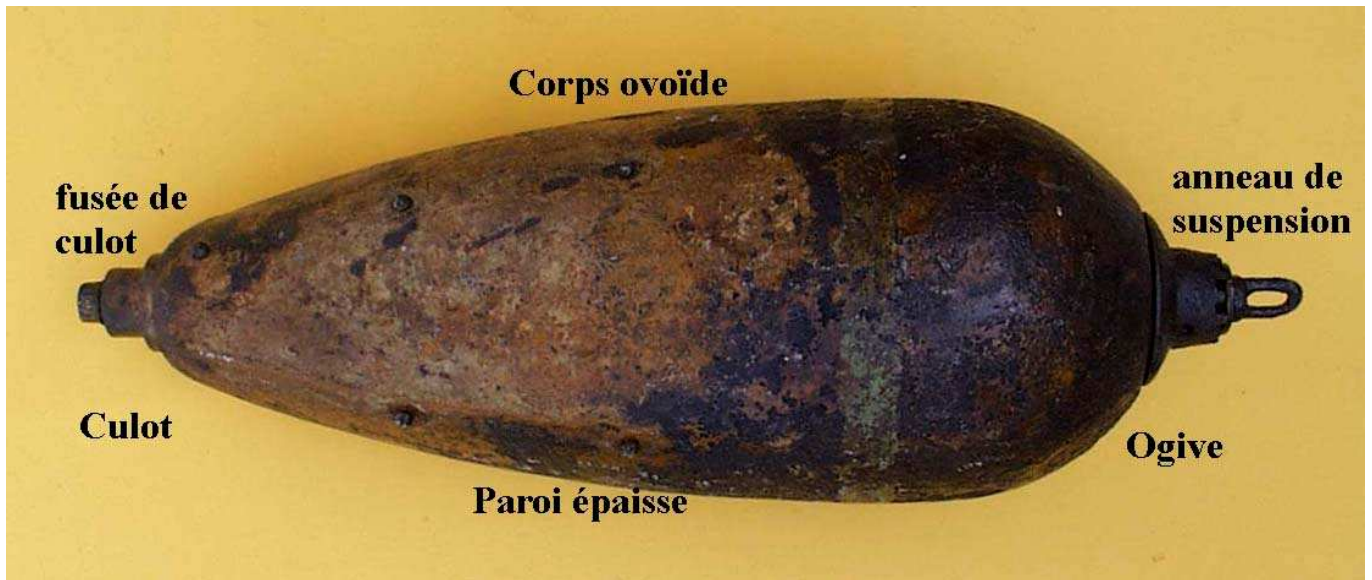
Bombe britannique de la première guerre mondiale
