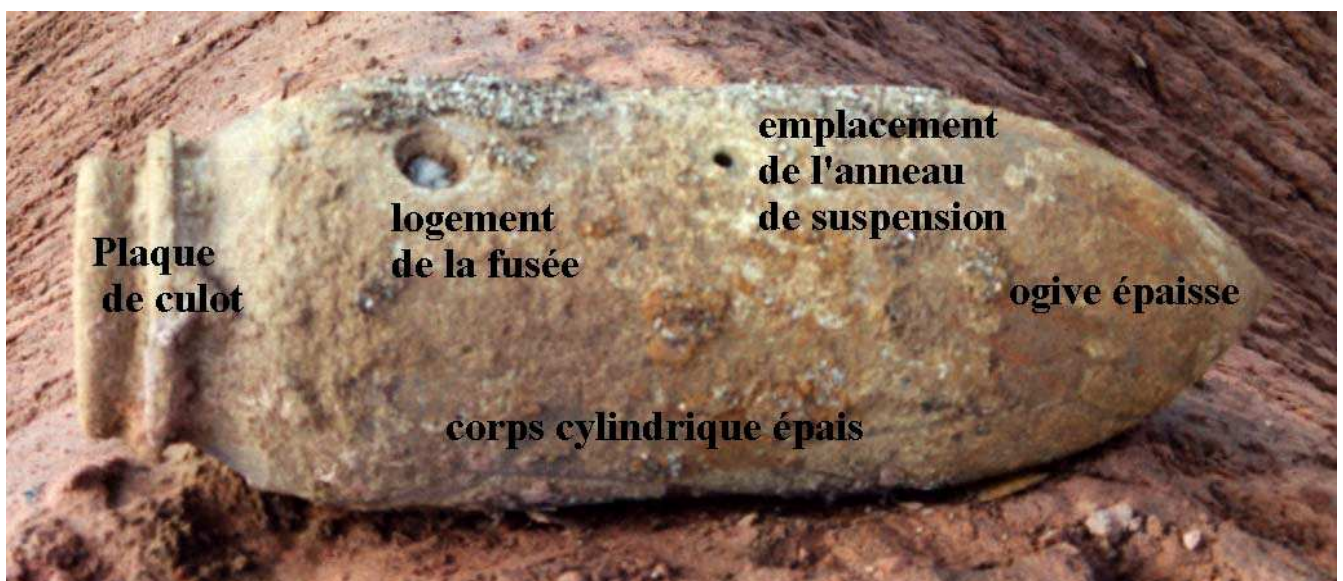
Bombe allemande à paroi épaisse de la seconde guerre mondiale type SD 500
