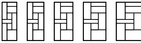
Šířka 800 mm
