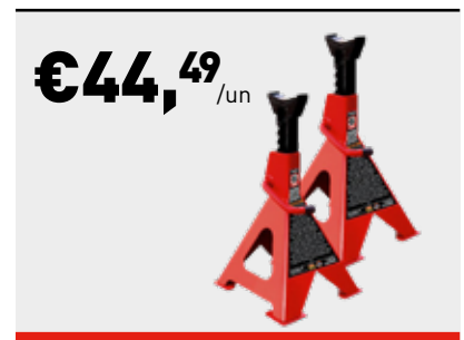
AB530000500 CAVALETE 6TON Altura mínima: 395 MM Altura máxima: 605 MM Peso N/B: 12,9 / 13,7 Kg
