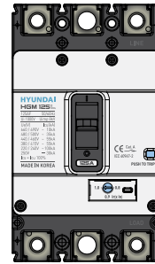
MCCB
