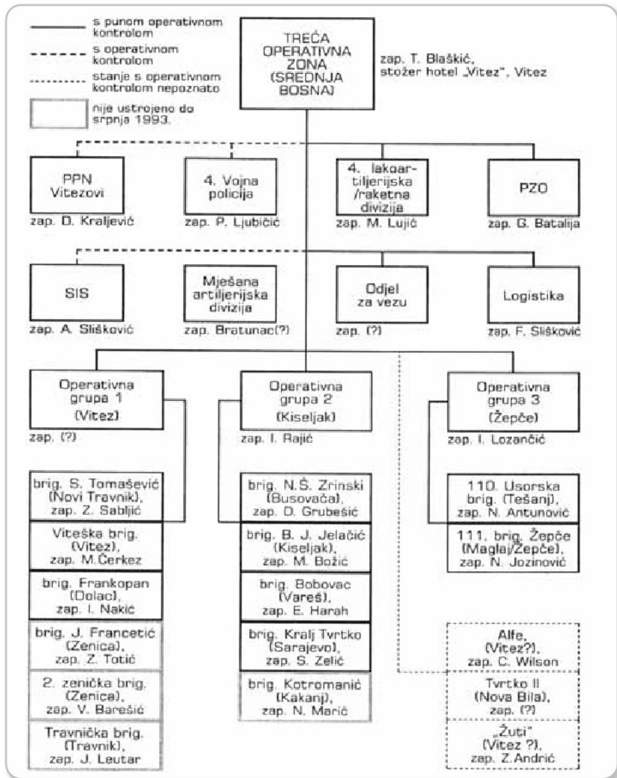
Shema: Treća operativna zona HVO
