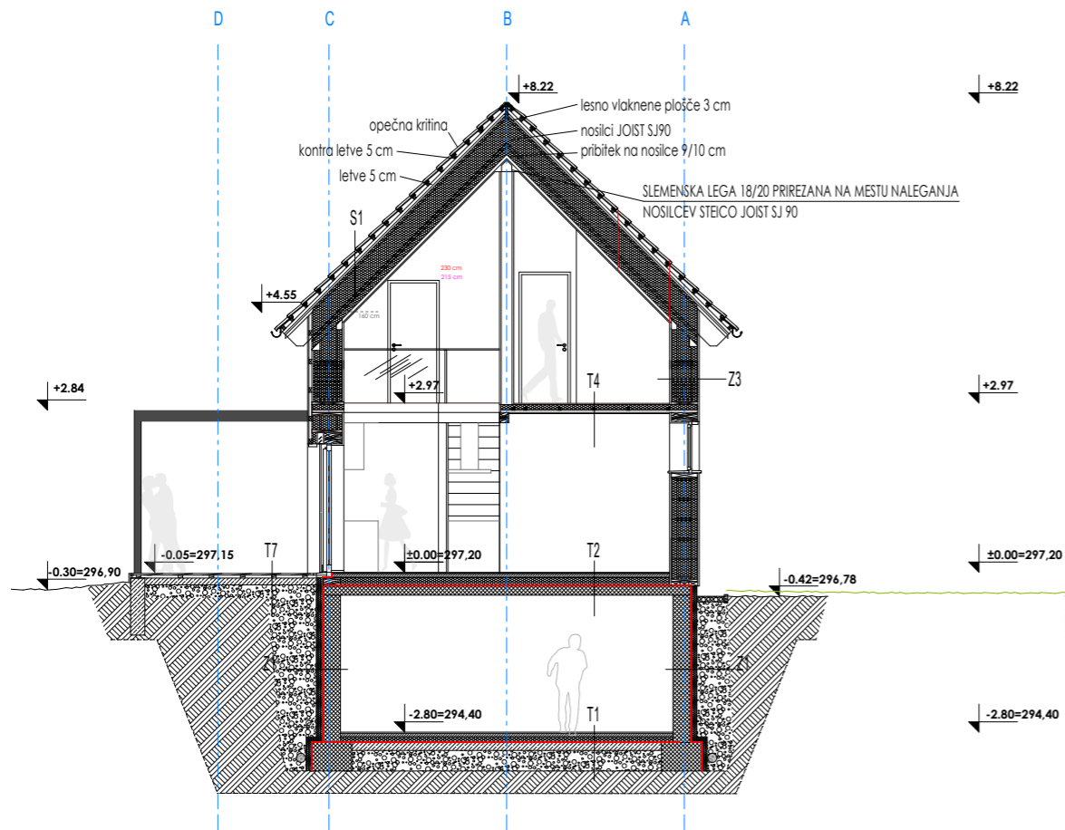
PREREZ A-A
