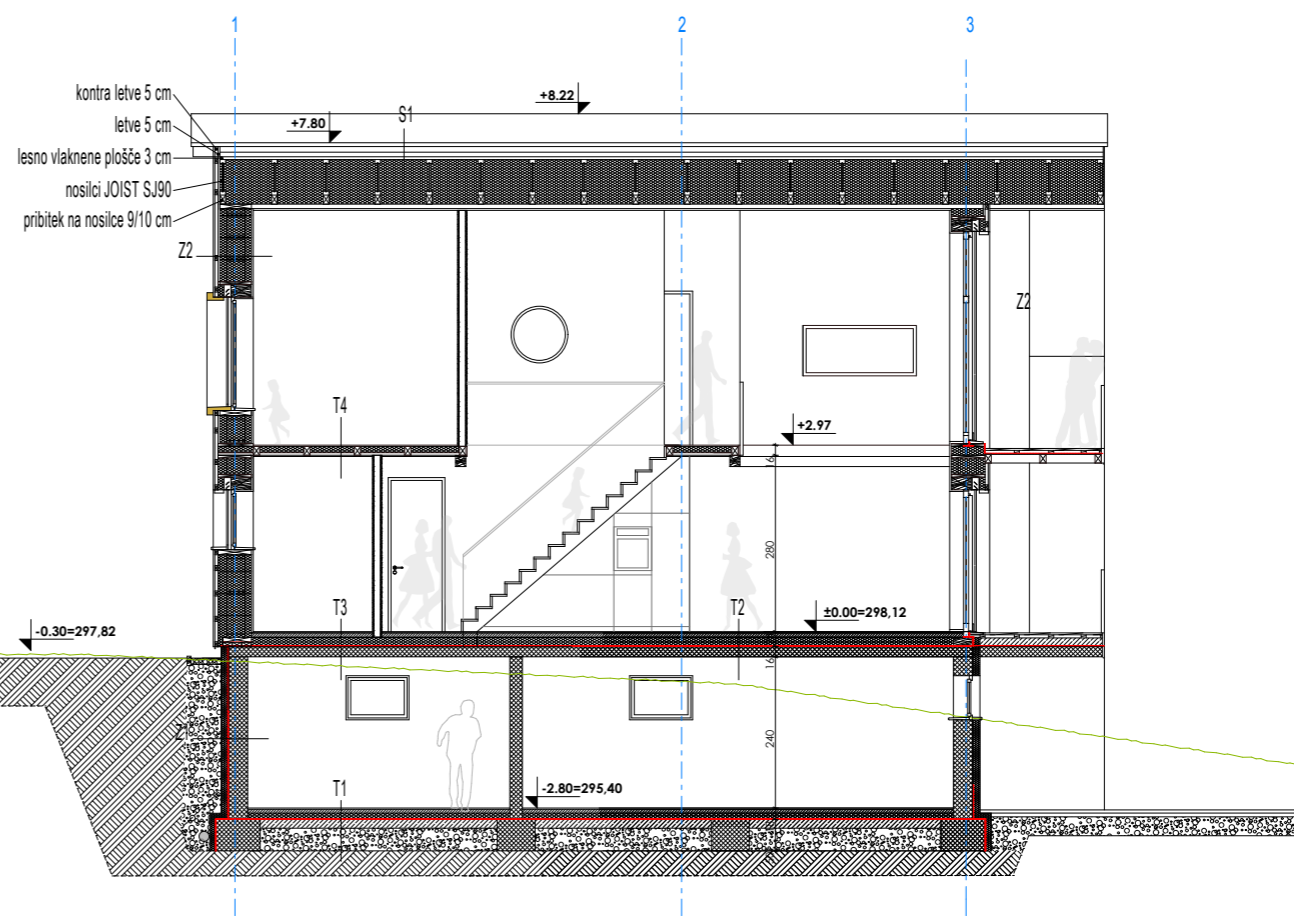
PREREZ B-B
