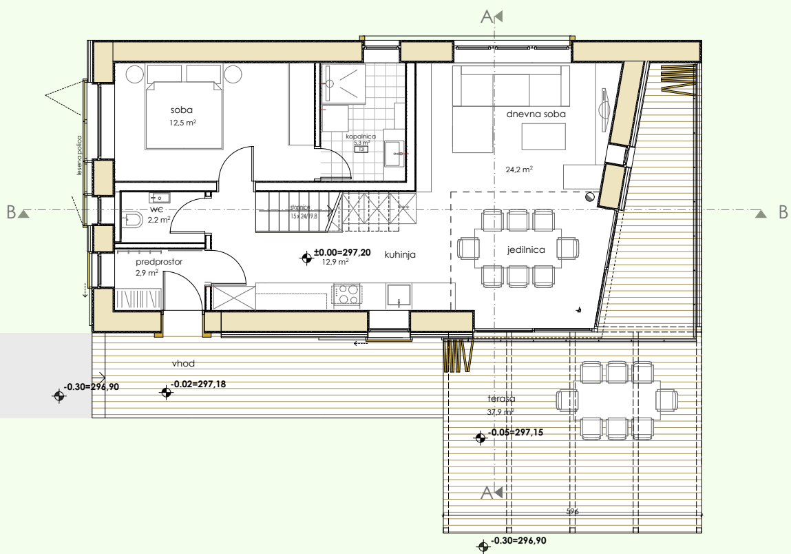
TLORIS PRITLIČJA
