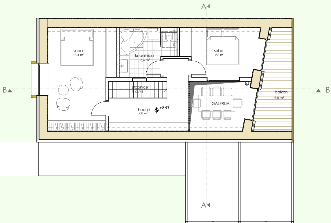
TLORIS MANSARDE
