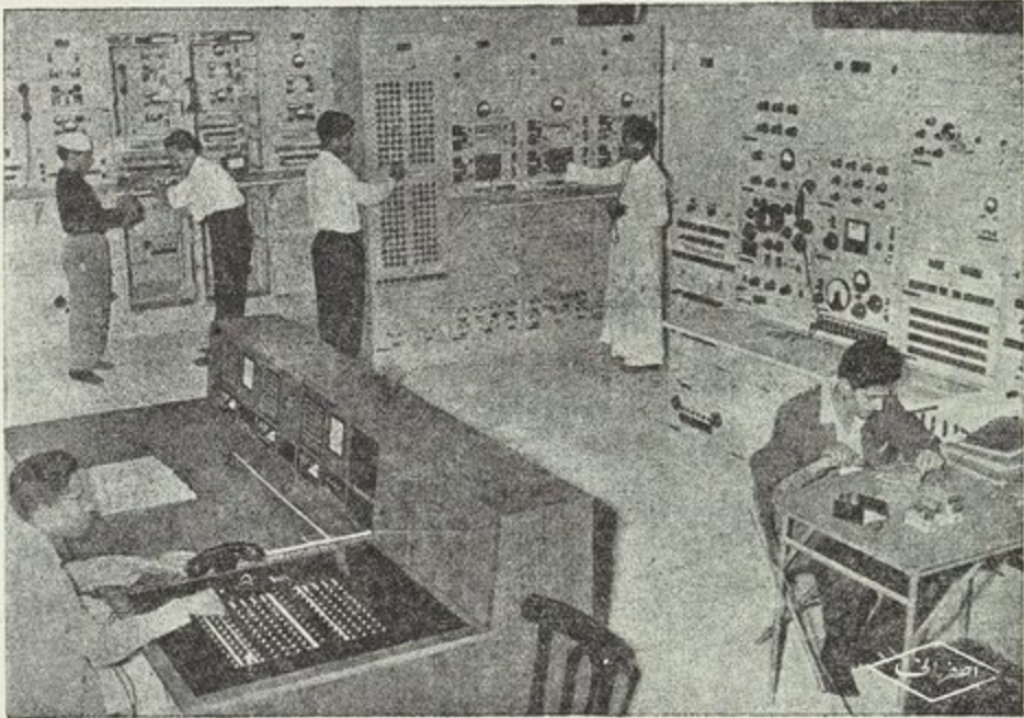
مراقبة شبكة الاتصالات التليفونية الاسلكية
