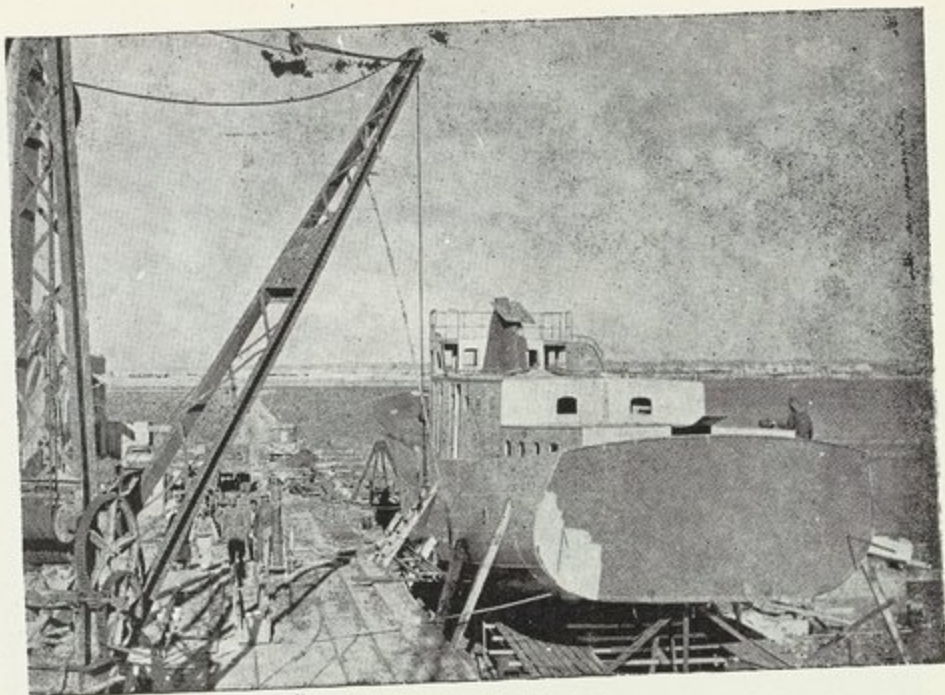
ترسانة بحرية لاصلاح وصناعة السفن الصغيرة ويرى احد الطرادات أثناء بنائه
