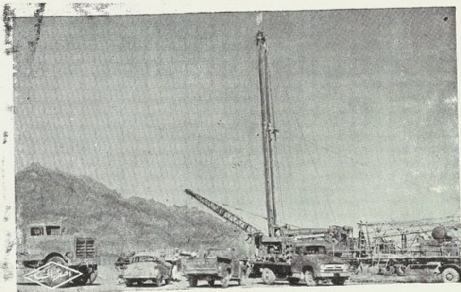
الاستعدادات الضخمة لعمال حفر الآبار بالمدينة المنورة
