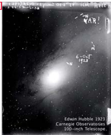
Historyczne zdjęcie Mgławicy Andromedy wykonane przez Hubble’a w nocy z 5 na 6 października 1923 r. Odkryta wtedy cefeida znajduje się między kreskami obok napisu „VAR!”.
