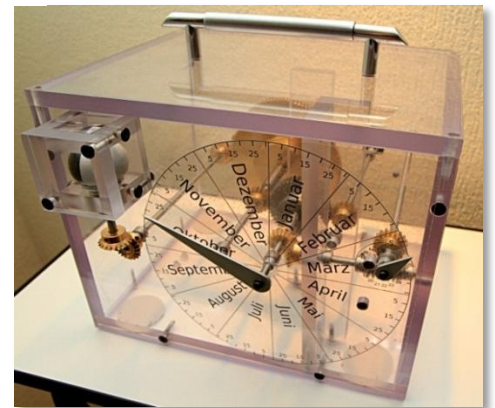
Der Antikythera-Mondphasencomputer
