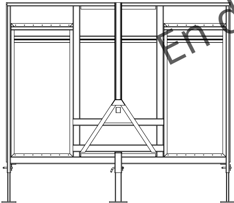
DÉTAIL A ECHELLE 1 : 10
