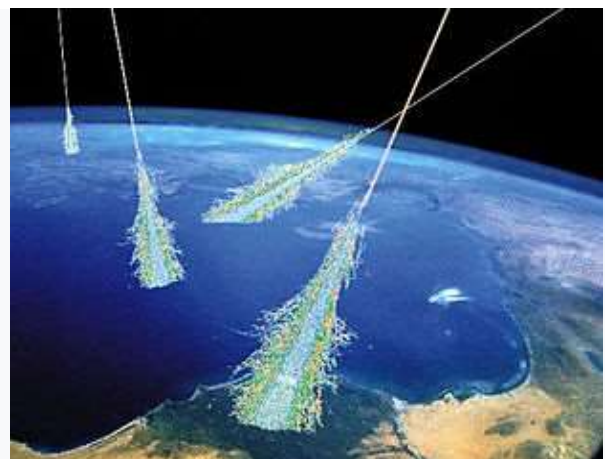
Interazione dei raggi cosmici con la troposfera
