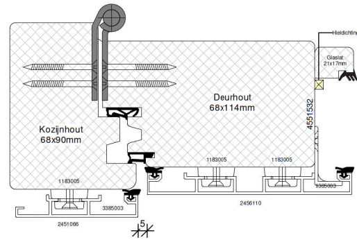
Droog beglazen (verdekt genageld)
