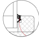
Droeg beglazen (verdekt genageel)
