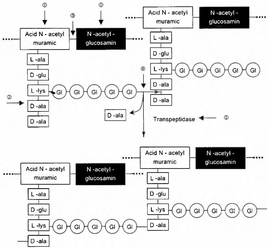
Hình 7.2. Sự hình thành peptidoglycan và vị trí tác động của các kháng sinh ức chế tổng hợp vách tế bào vi khuẩn: ① Fosfomycin; ② Cycloserin; ③ Bacitracin; ④ Vancomycin; ⑤ Các \beta - lactam.
