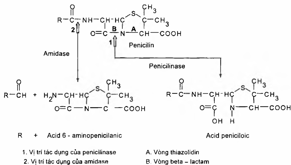
Hình 7.6. Công thức của penicilin và vị trí tác động của enzym phân huỷ thuốc
