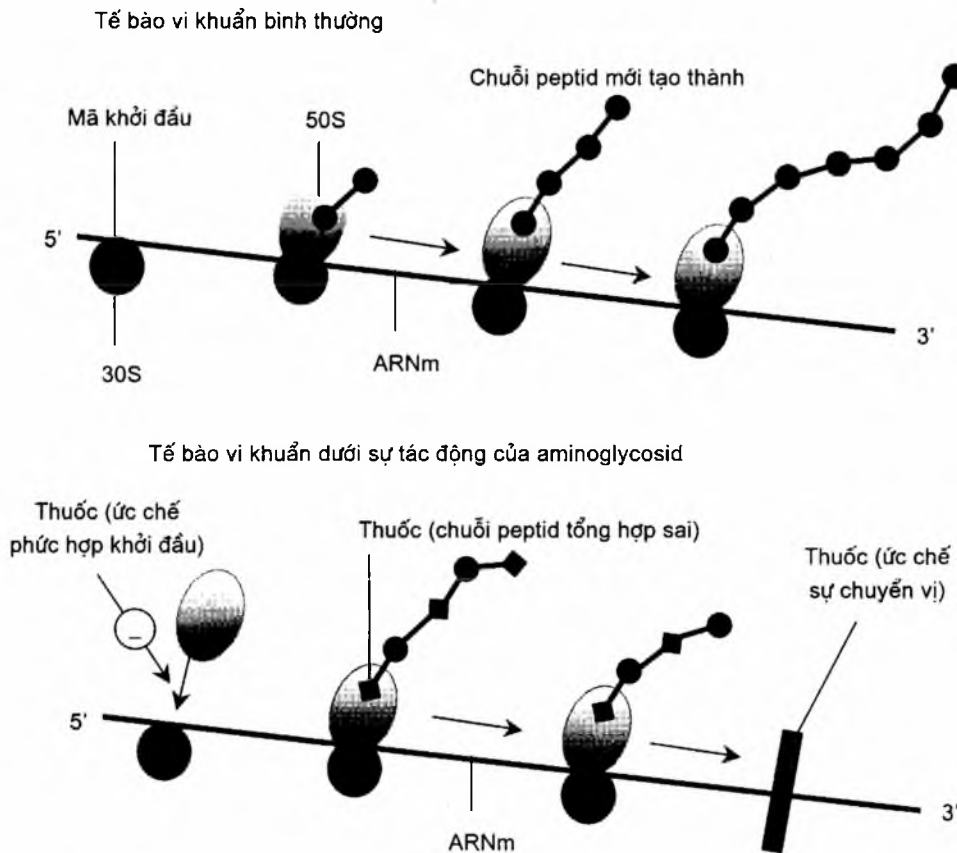
Hình 7.4. Cơ chế tác dụng của aminoglycosid
