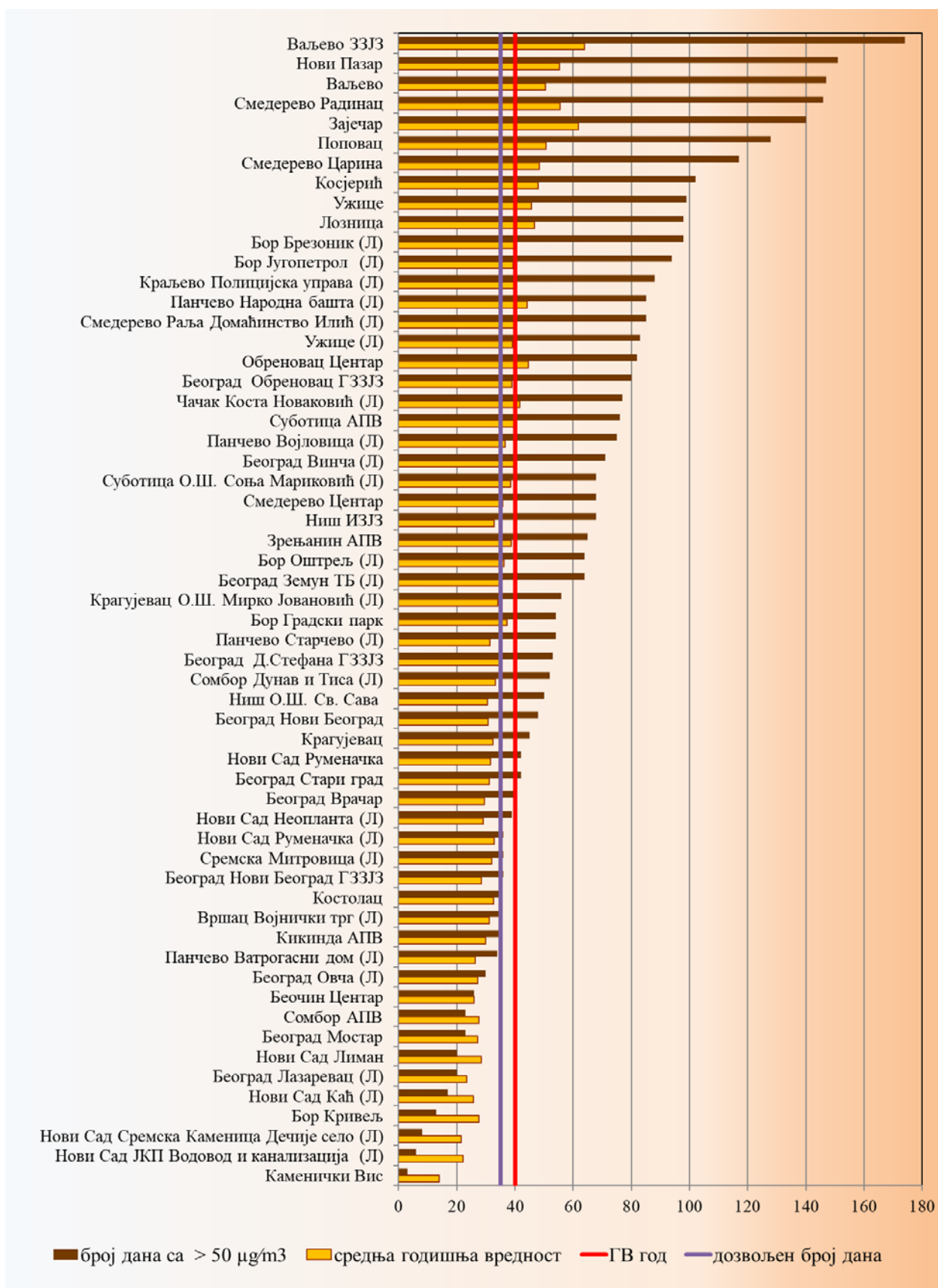
Слика 10. Упоредни приказ средње годишње концентрације PM_{10} ( \mu g/m^3 ) и броја дана са прекорачењем ГВ у 2021. години
