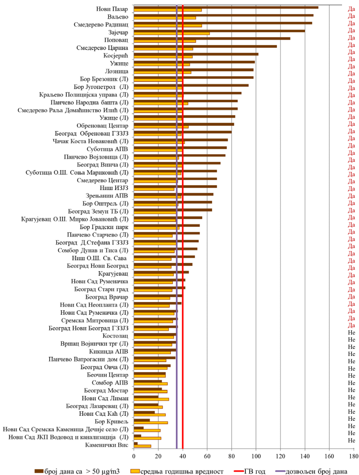
Слика 23. Упоредни приказ средње годишње концентрације PM_{10} ( \mu g/m^3 ), броја дана са прекорачењем ГВ у 2021. години и обавезе израде планова квалитета ваздуха
