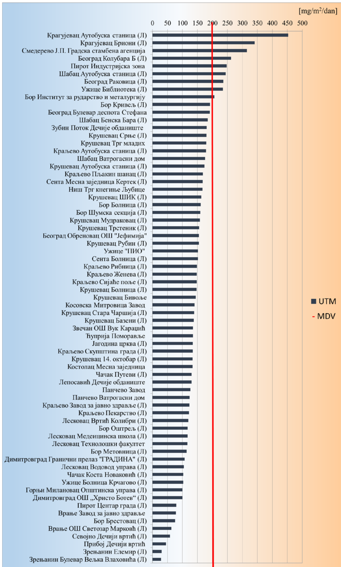
Слика 32. Средња годишња вредност укупних таложних материја (mg/m 3 /dan) у 2021. години и максимална дозвољена годишња вредност (mg/m 3 /dan)
