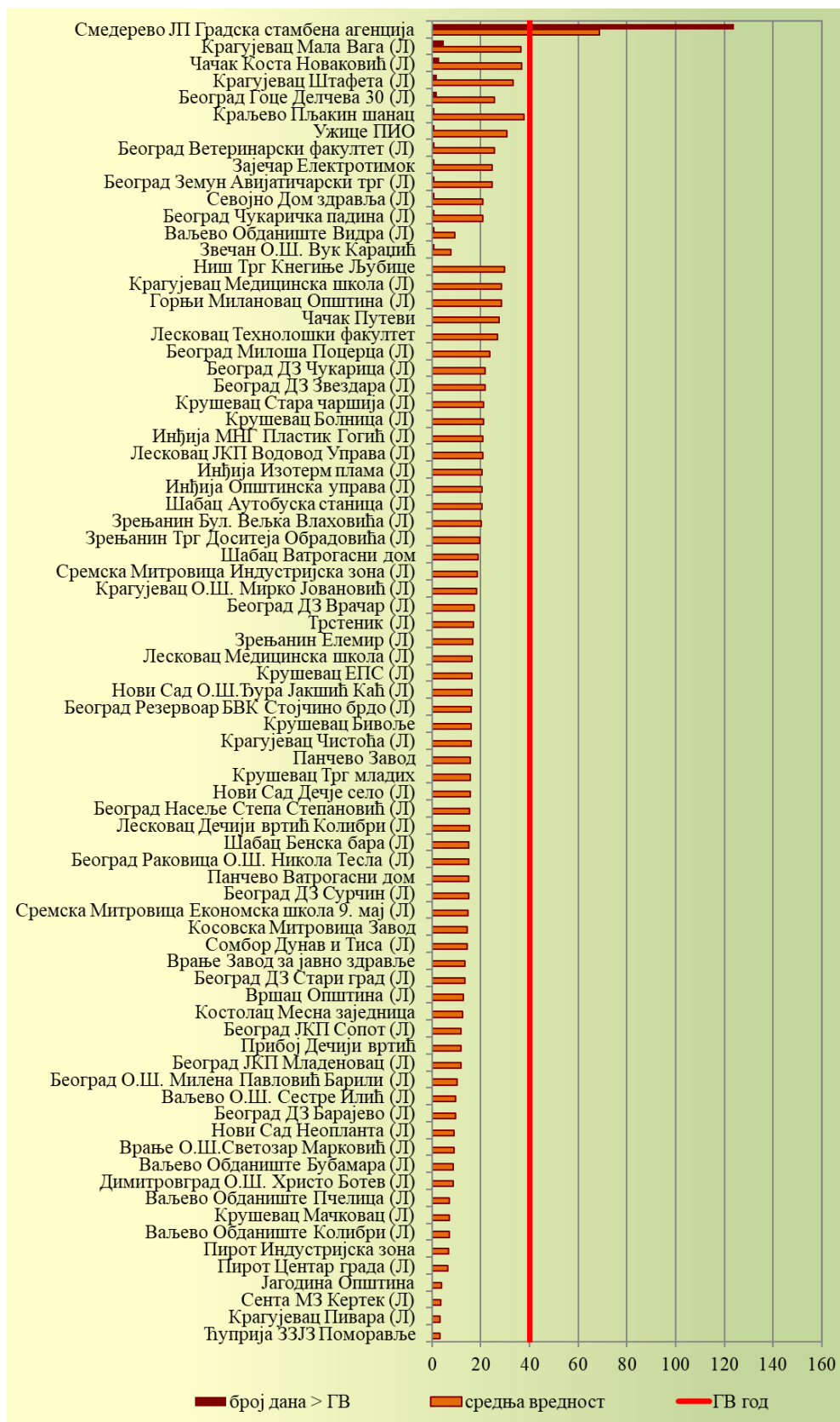
Слика 30. Средња годишња концентрација NO 2 (µg/m 3 ) и број дана са прекорачењем ГВ у 2021. години
