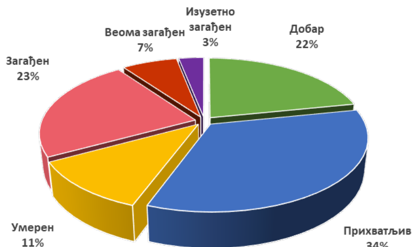
Слика 26. Расподела учешћа различитих индекса квалитета ваздуха за PM_{2.5} у Београду, према критеријумима ЕЕА, у 2021. години
