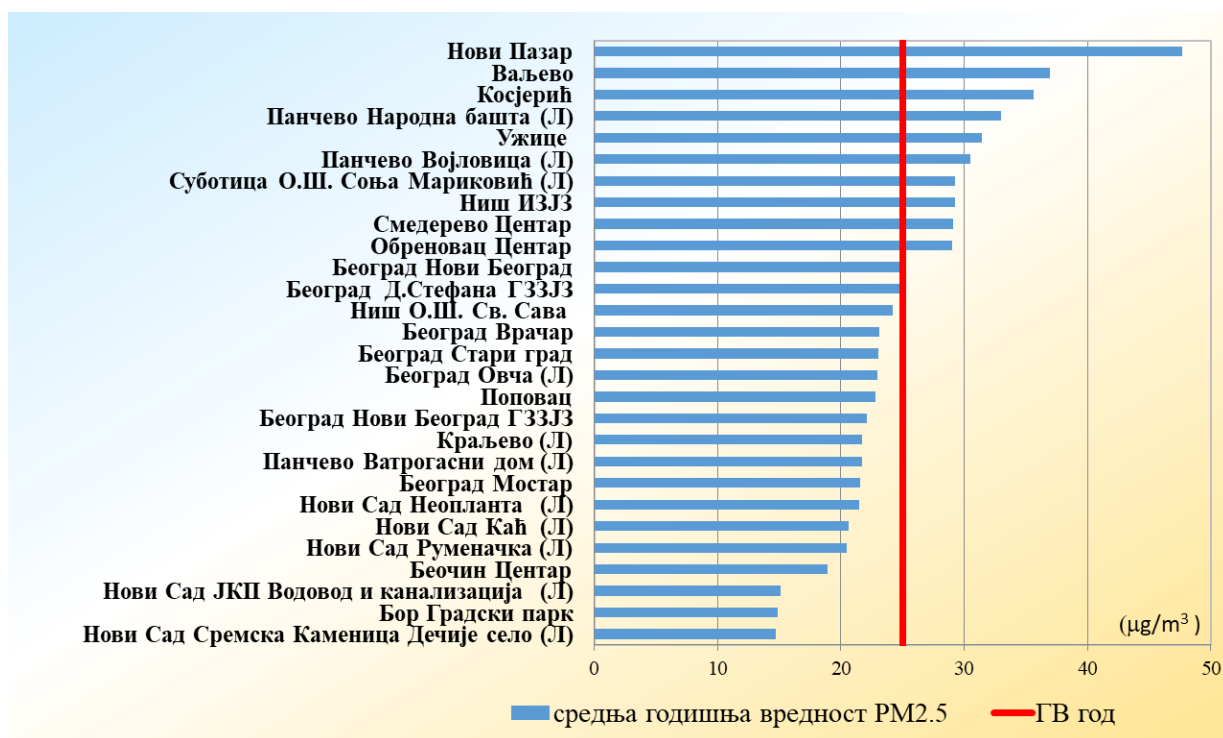
Слика 13. Средње годишње вредности PM 2.5 (µg/m 3 ) у 2021. години
