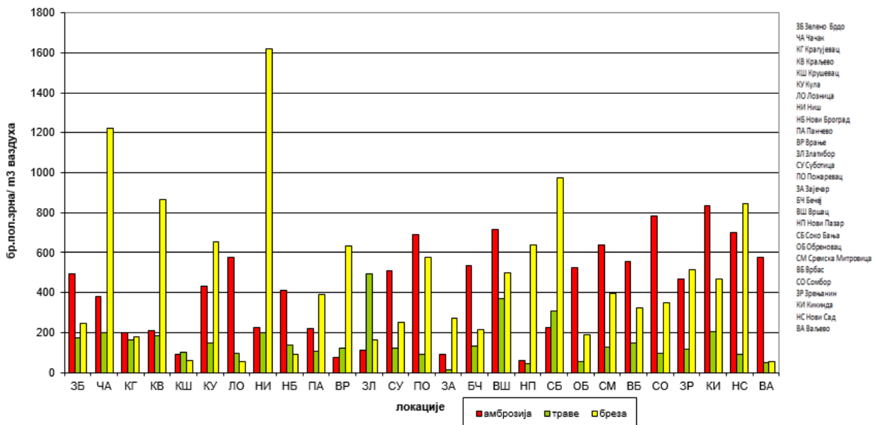
Слика 34. Максимална концентрација поленових зрна на свим станицама у Републици Србији у 2021. години
