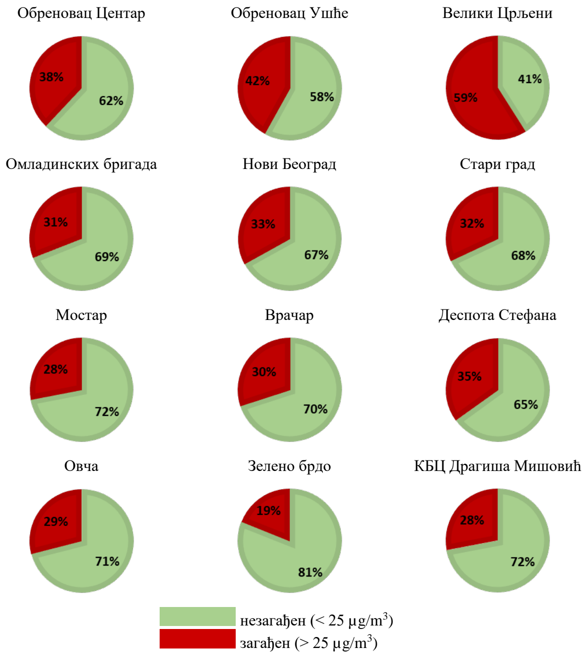
Слика 28. Расподела индекса квалитета ваздуха за \text{PM}_{2.5} у категоријама загађен (црвено) и незагађен (зелено) за мерна места у Београду у 2021. години (види слику 25.б)
