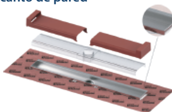
TECEdrainline-Evo Canaleta de ducha con canto de pared
