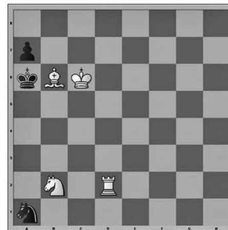
Ход белых. Мат в 2 хода. White's move. Mate in 2.
