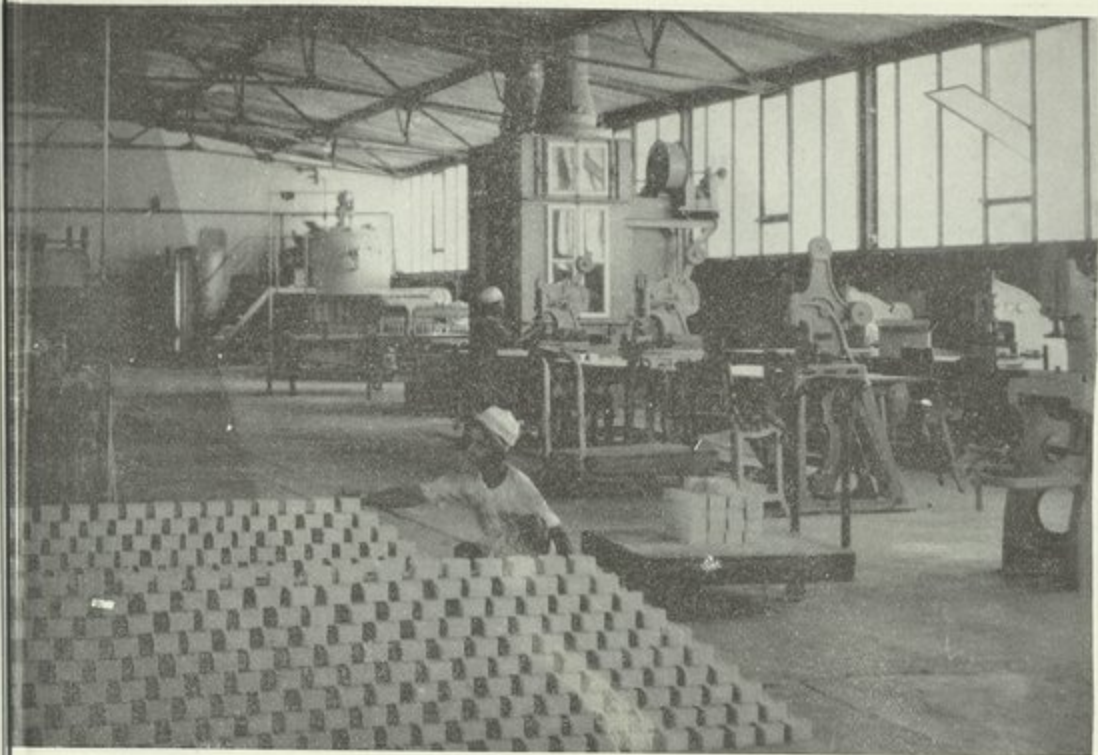
صناعة الطوب العازل للحرارة
