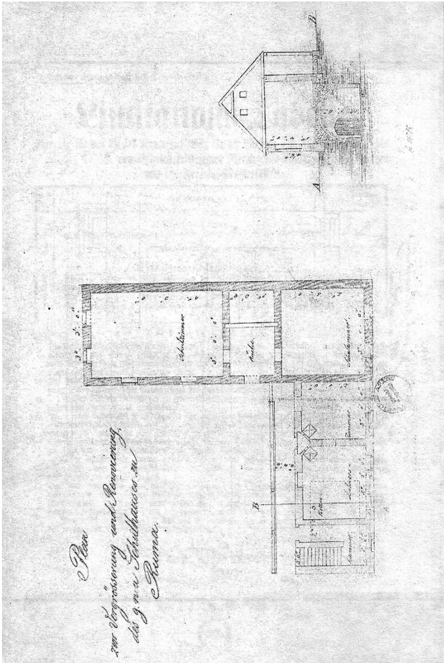
Plan za dogradnju i renoviranje zgrade srpske škole, 1858. godina (IAS, Sr. Mitrovica, Fond – Magistrat trgovišta Ruma)
