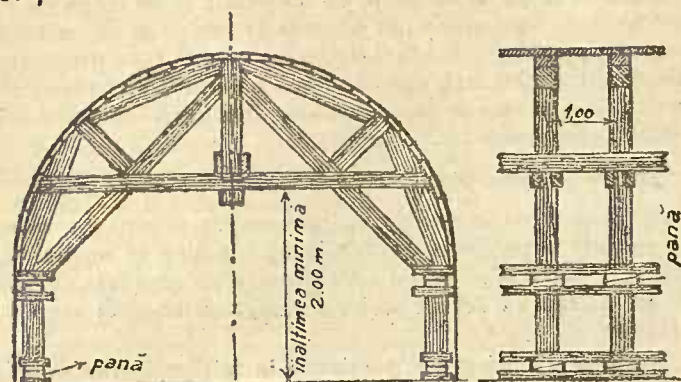
Sustinerea bolților pivnițelor Secțiune transversală. Secțiune longitudinală.
