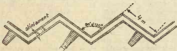
Fig. 12. Șanț-adăpost în cremalieră, în teren bun. E suficient de a da șanțului o lărgime de 0,80 m la fund și de 1,40 m la suprafață.
