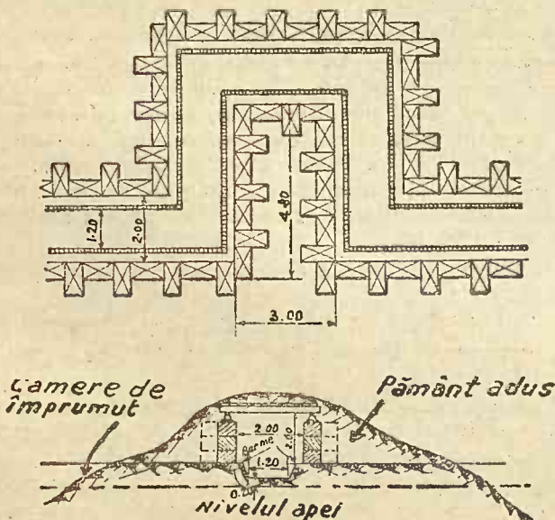
Fig. 13. Șanț-adăpost de suprafață, cu traverse și căptușit cu cutii, având dimensiunile de 1 m pe 0,50 m.
