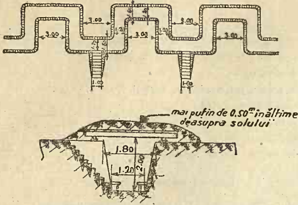
Fig. 11. Șanțuri-adăpost cu traverse în teren bun. În acest model de tranșee pot încăpea 4 persoane pe metru curent.
