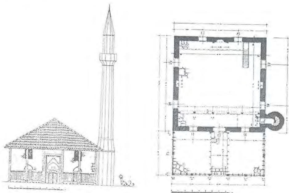
Fasada i tlocrt džamije na Ustikolini (nacrt ing. E. Dimitrijević, 1955.)
