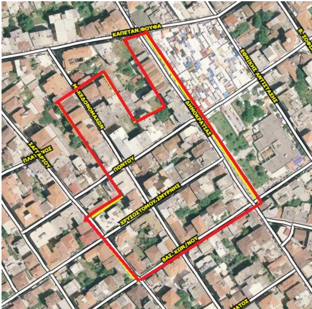
Περίγραμμα των οδών διακοπής Ρεύματος
