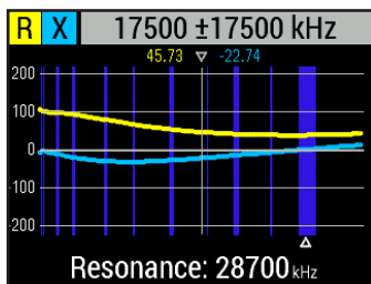
Beispiel 2: Unknown Kabel
