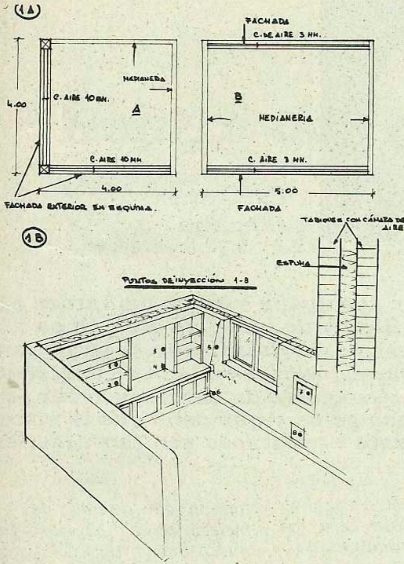
En el dibujo (1 A) se observa que el volumen de cámara de la vivienda A es más del doble que el de la B.
