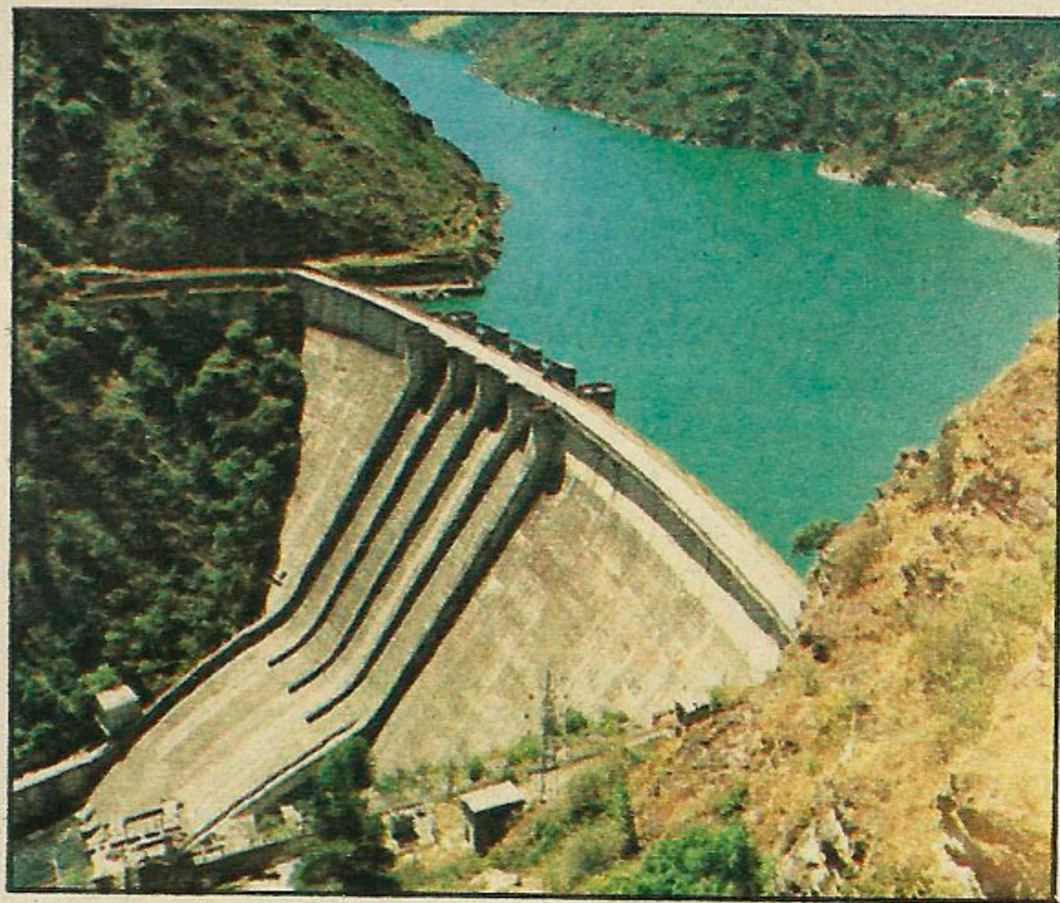
EMBALSE FRAUDAS DE SALIME.
