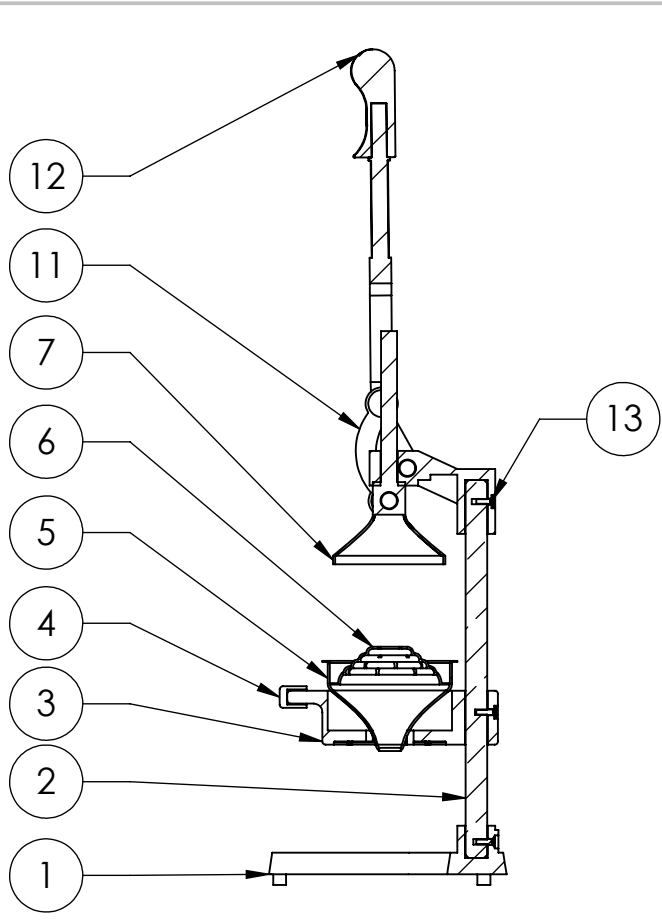
SECTION A-A
