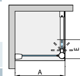
FUD2 + stabilizační vzpěra
