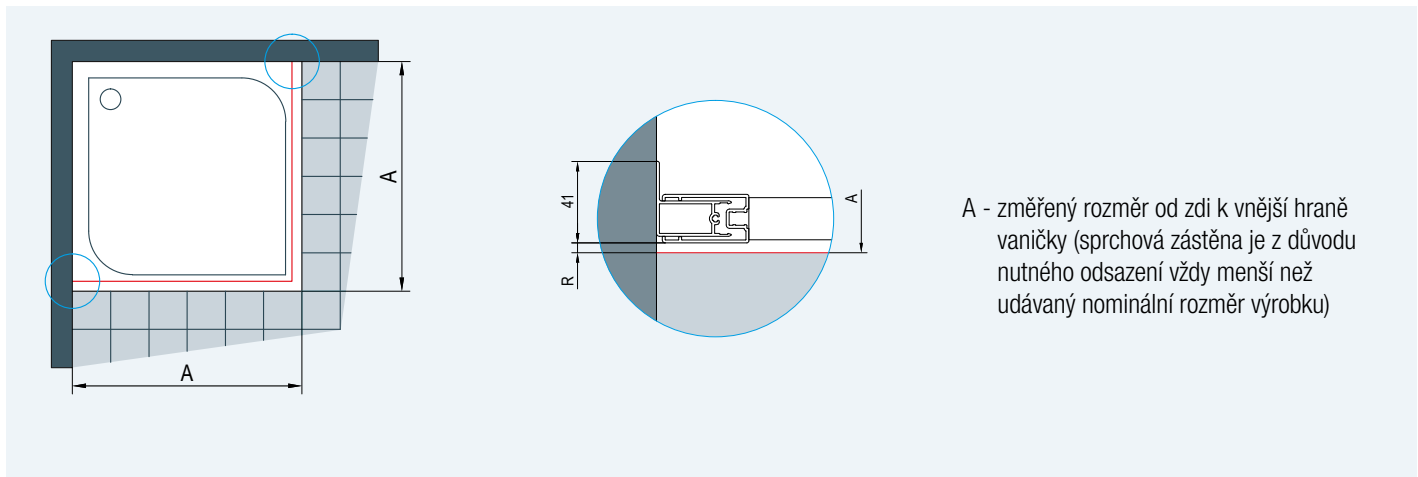
Obr. 1: Při montáži na vaničku je odsazení R (viz detail 1) závislé na velikosti rádiusu vnější hrany vaničky a je stejné pro standardní i zvláštní rozměry.
