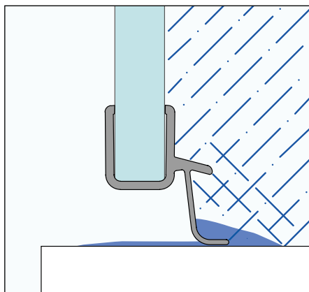
Bezrámové zástěny bez prahové lišty
