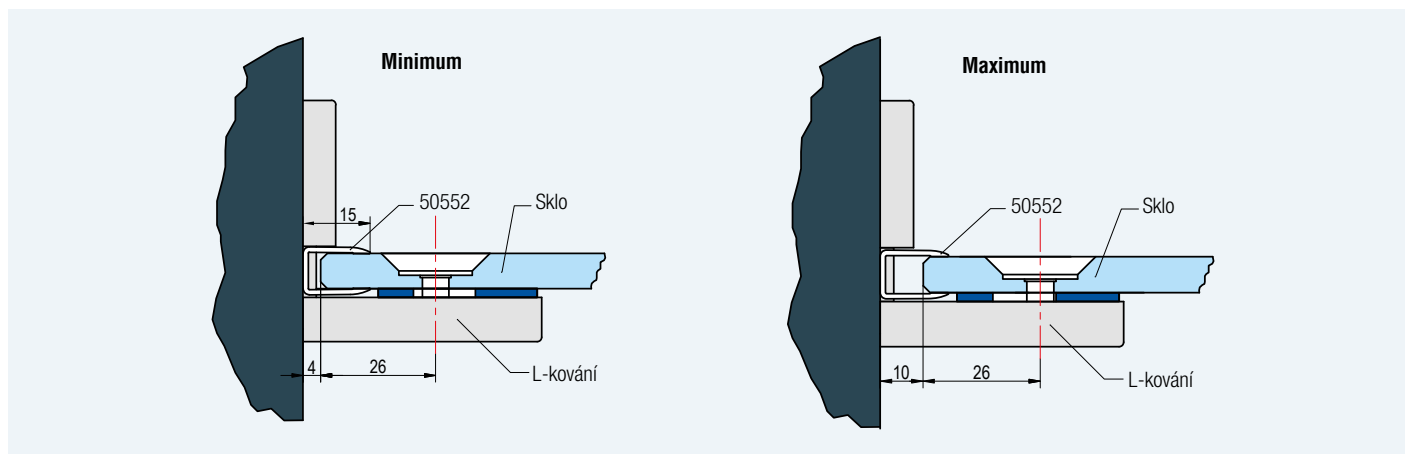
Obr. 5: L-kování s těsnicím U-profilem 50552 umožňuje vyrovnání nerovností zdi do 6 mm. Těsnicí U-profil 50552 umožňuje zakrýt mezeru mezi zdí a sklem.
