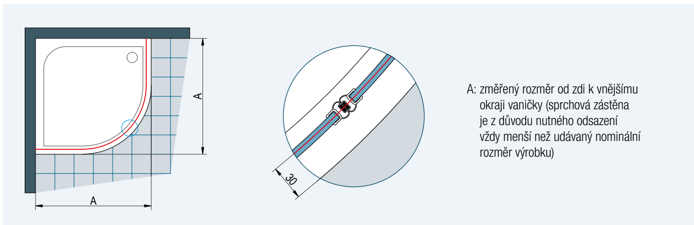
Obr. 3: Při montáži na vaničku je odsazení 30 mm stejné pro standardní i zvláštní rozměry.
