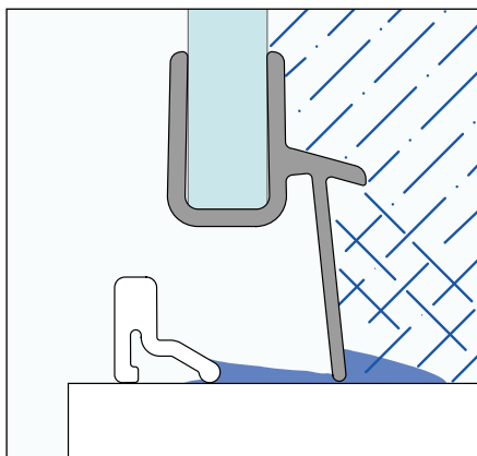
Částečně rámové zástěny s prahovou lištou
