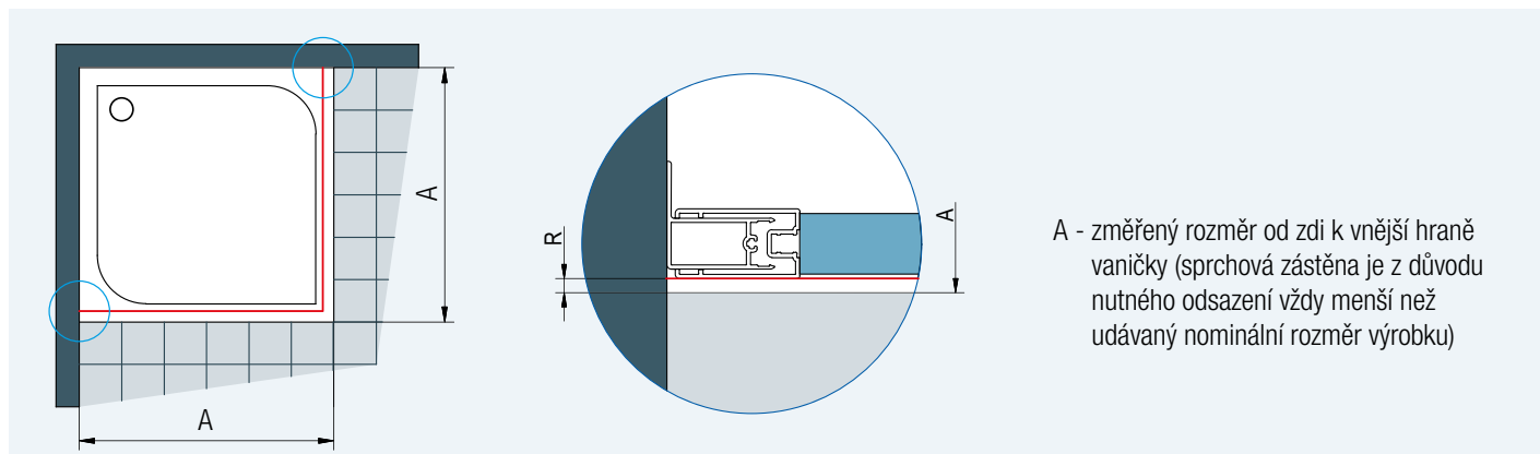
Obr. 1: Při montáži na vaničku je odsazení R (viz detail 1) závislé na velikosti rádiusu vnější hrany vaničky a je stejné pro standardní i zvláštní rozměry.
