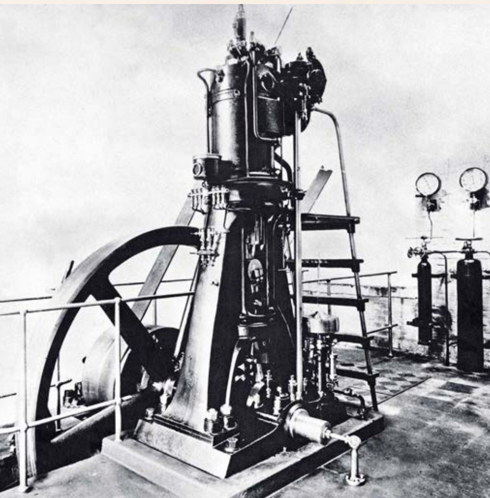
Pierwszy silnik wysokoprężny zbudowany w fabryce Kruppa w 1897 r.
