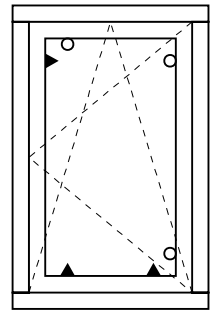
draaival ramen
