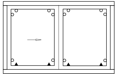
horizontaal schuifraam/deur
