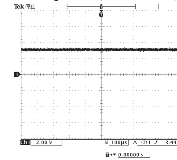
POINT ⑦ XL502 (Pin 12 of IC504)
