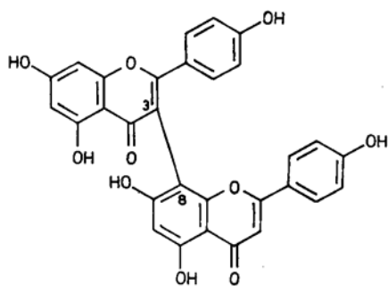
13,118-Biapiigenin
