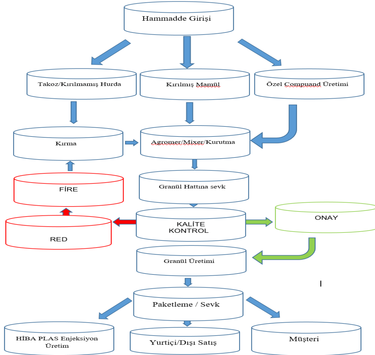
5.1: Plastik Granül Extruder ve Kırma Ünitesi İş Akım Şeması
