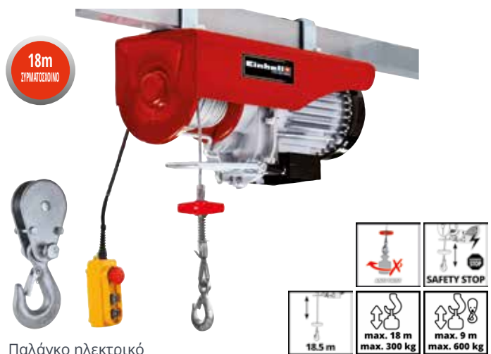
Παλάγκο ηλεκτρικό
