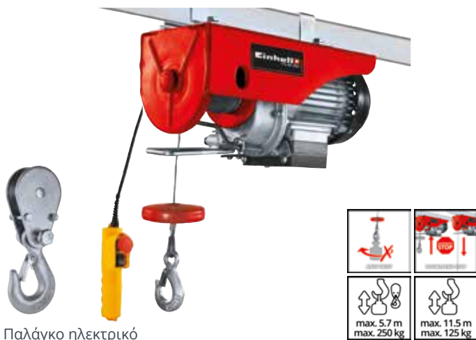
Παλάγκο ηλεκτρικό
