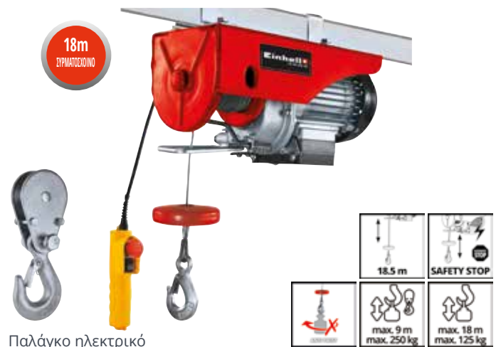
Παλάγκο ηλεκτρικό
