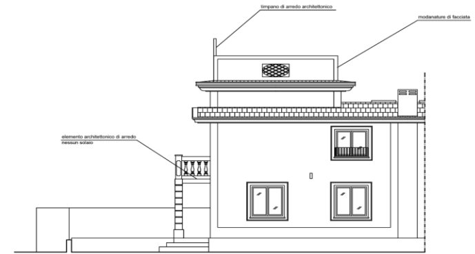
PROSPETTO LATERALE DESTRO
