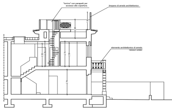
SEZIONE A-A
