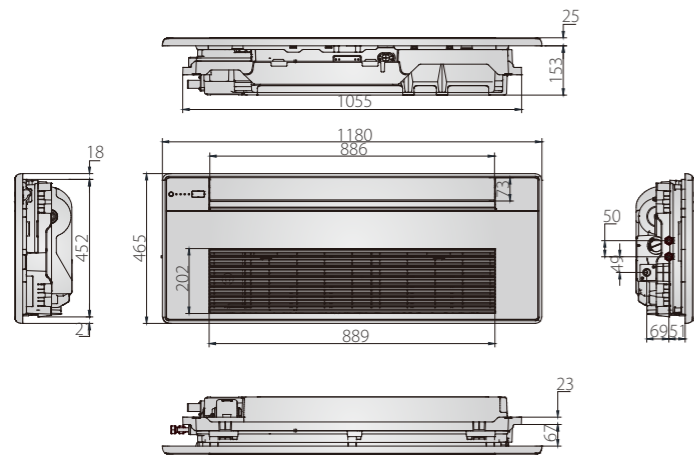
MKC-V300R-B
