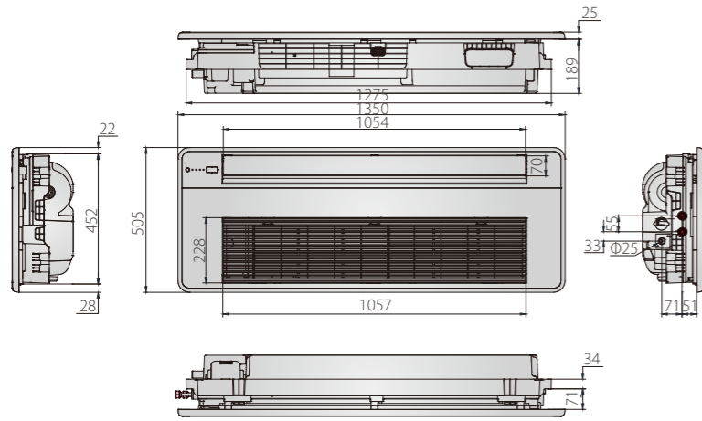
MKC-V400R-B MKC-V600R-B
