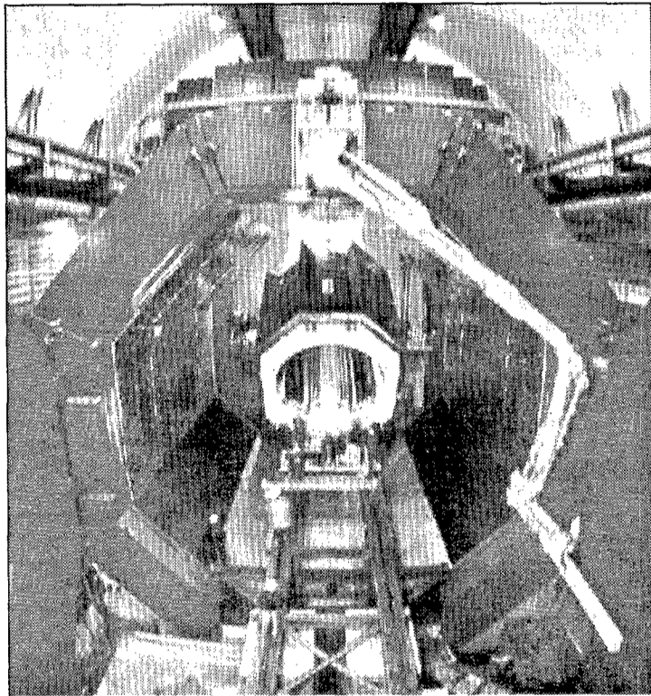
Túnel del acelerador de partículas LEP situado en Ginebra (1990).
