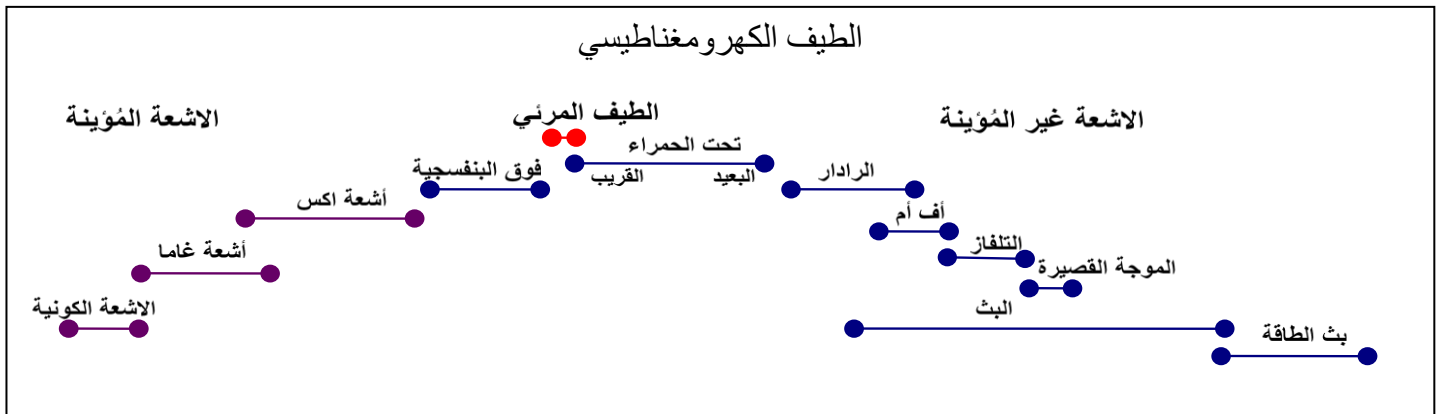
الشكل 12-1 الطيف الكهرومغناطيسي
