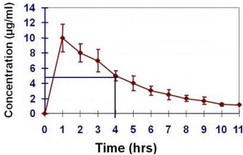
الشكل ٥-٢: وصف لمبدأ فترة نصف العمر
