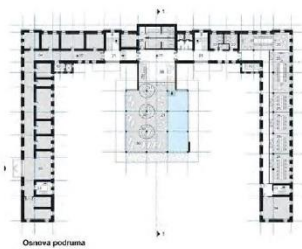
Osnova podzrmana
