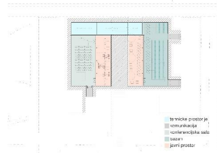
Osnova podruma - R 1:250
