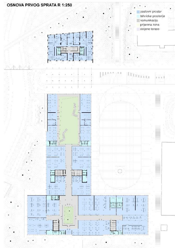
OSNOVA PRVOG SPRATA R 1:250
