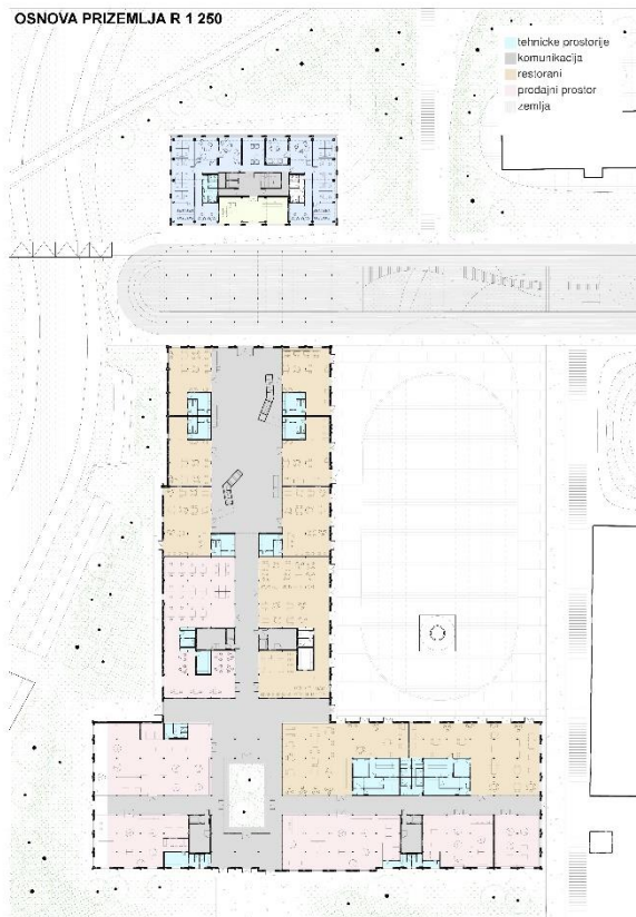
OSNOVA PRIZEMLJA R 1:250
