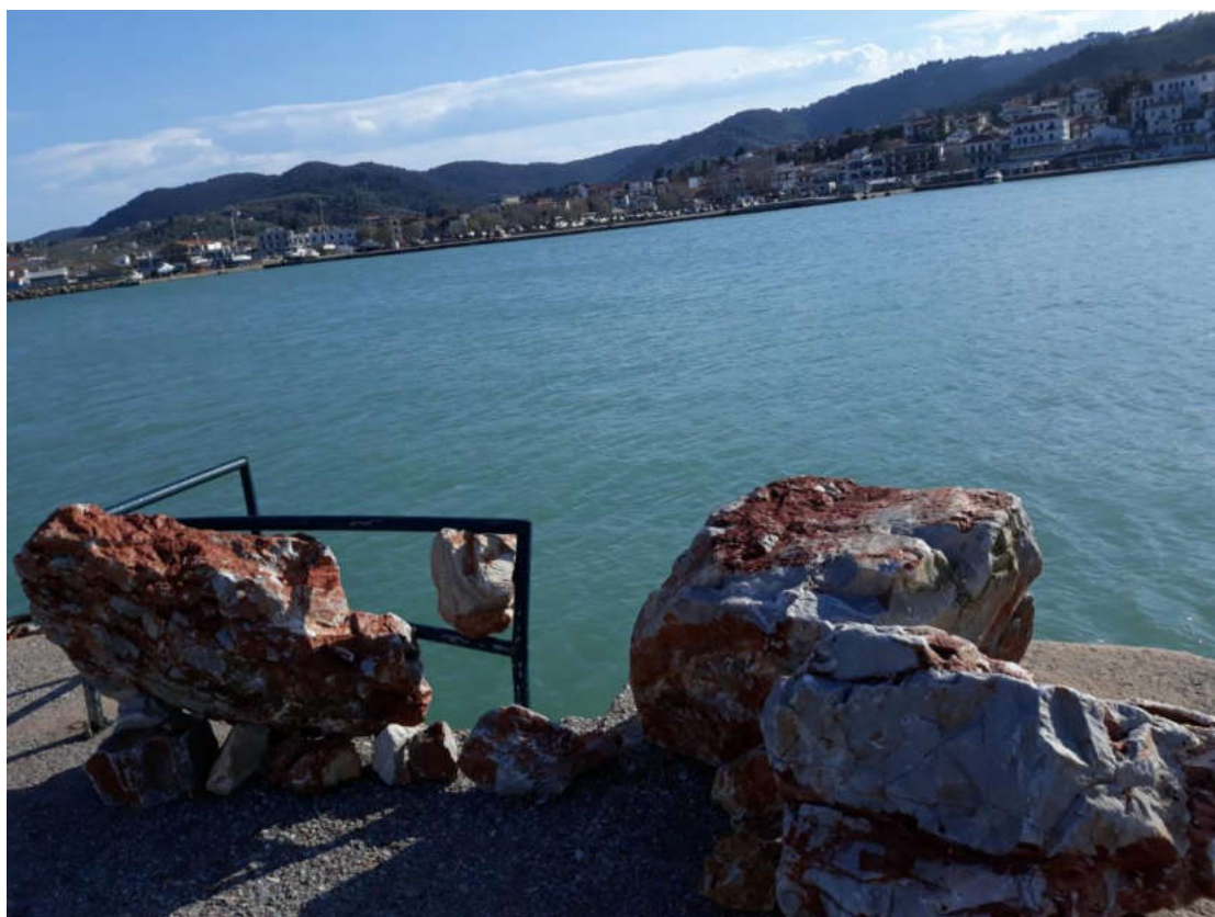
(ΛΙΜΑΝΙ ΣΚΟΠΕΛΟΥ)
