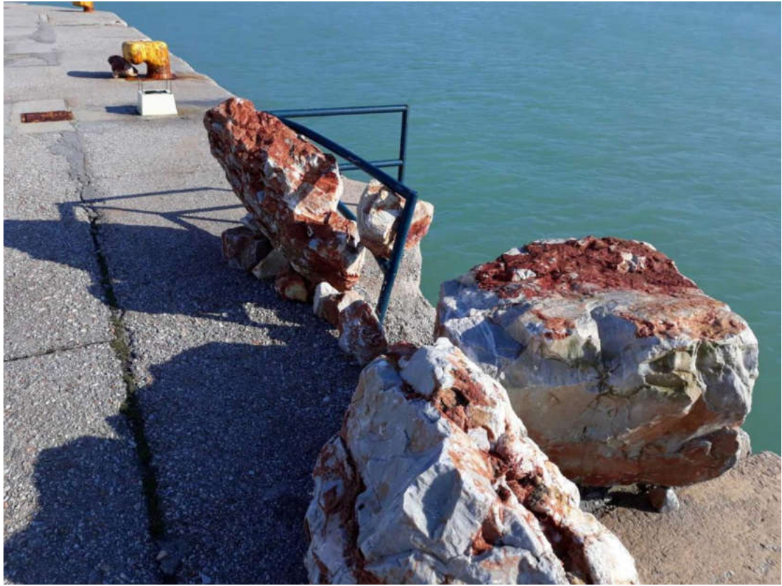
(ΛΙΜΑΝΙ ΣΚΟΠΕΛΟΣ)
