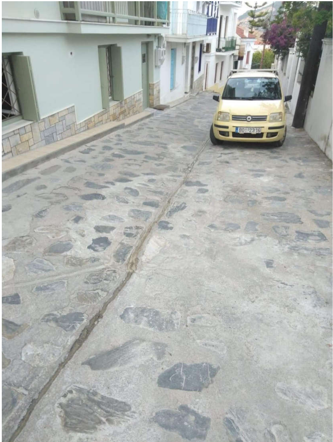
(Εργασίες αποκατάστασης πλακόστρωτου)
