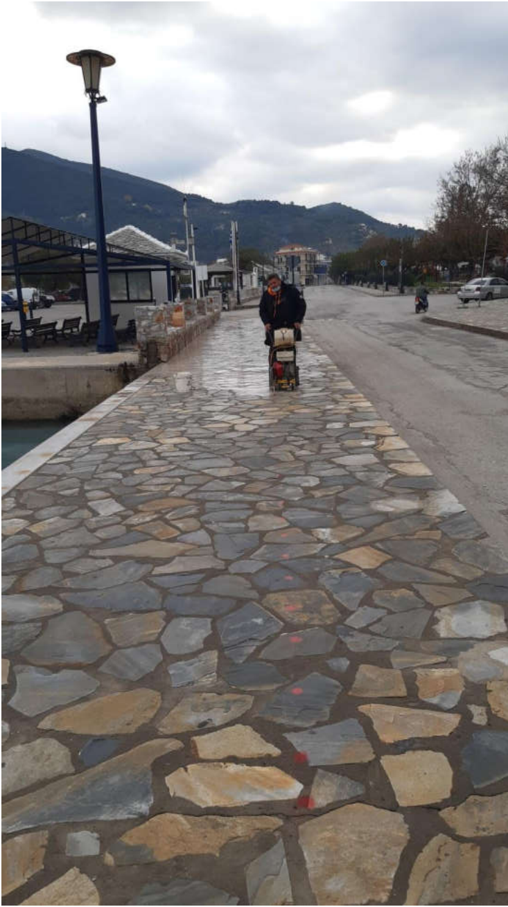
(Λιμάνι Σκοπέλου)
