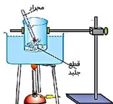
انصهار الجليد
