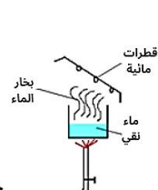
التبخير + التكاثف
