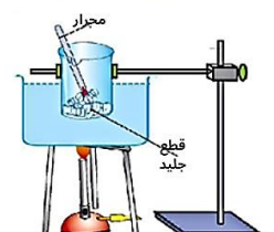
انصهار الجليد
