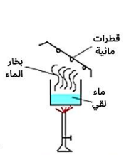
التبخير + التكاثف
