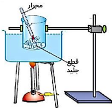
انصهار الجليد
