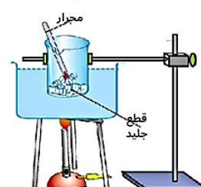
انصهار الجليد
