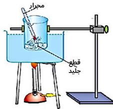
انصهار الجليد
