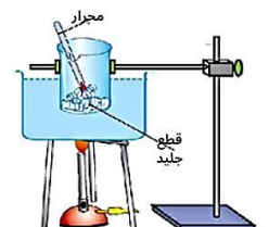
انصهار الجليد
