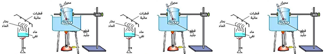
التبخير + التكاثف
