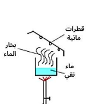
التبخير + التكاثف
