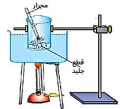
انصهار الجليد
