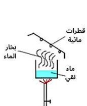
التبخير + التكاثف
