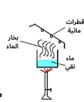
التبخير + التكاثف
