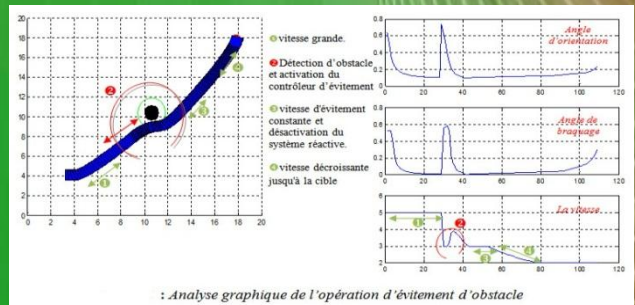
Analyse graphique de l'opération d'évitement d'obstacle
