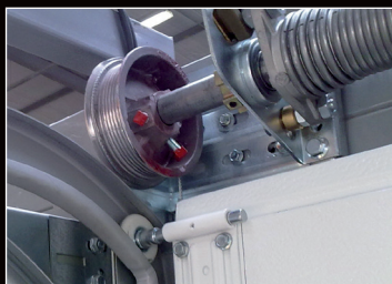
Rampe de ressorts galvanisés adaptée au poids de la porte.
