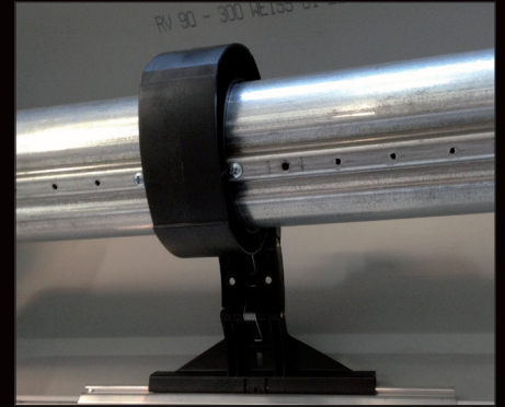
Verrou automatique anti-souèvement Retardateur d'effraction
