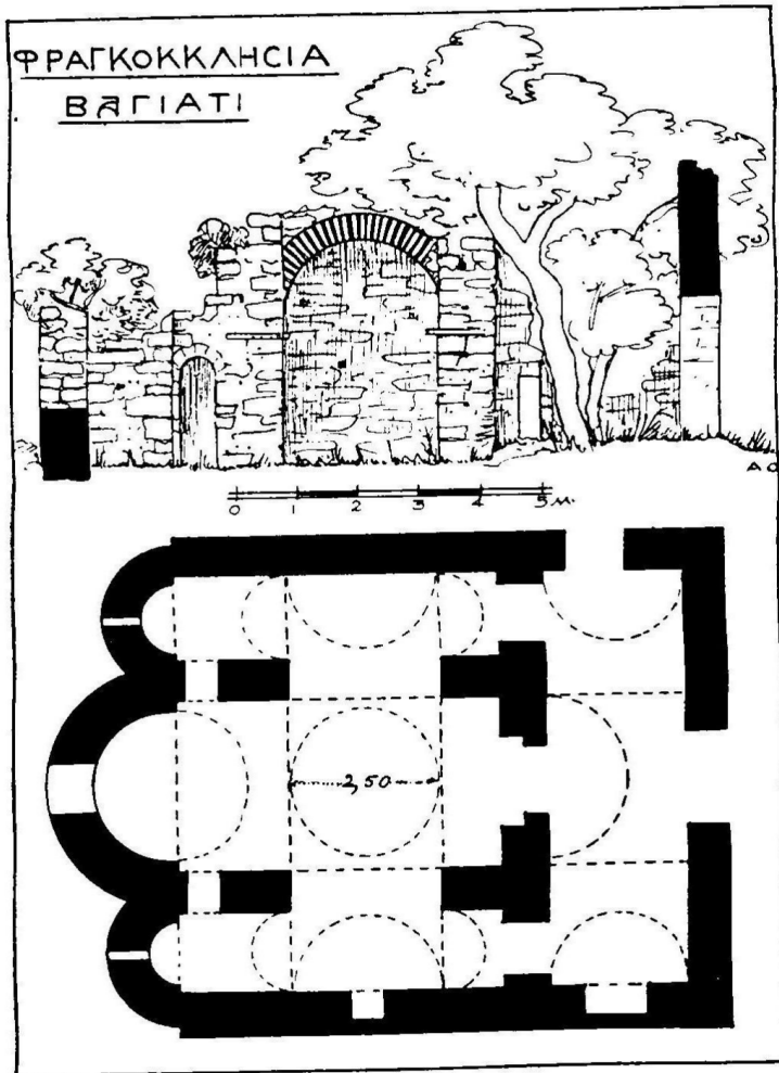
Εἰκ. 259. Κάτοψις καὶ τομὴ τῆς Φραγκόκκλησιαις.
