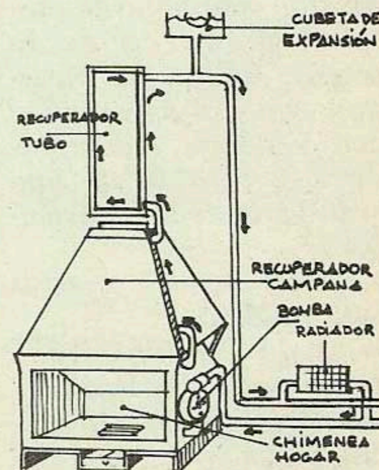
B: Sistema de recuperación de calor extensible a toda la casa.
