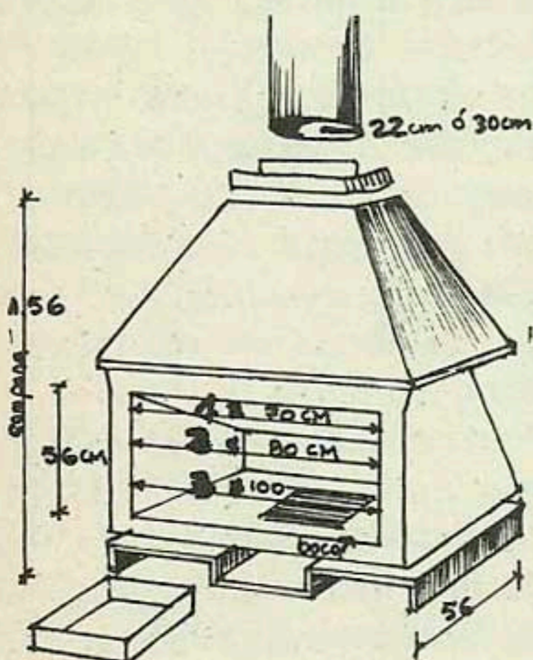
C: Medidas distintas de boca y campana de la chimenea.
