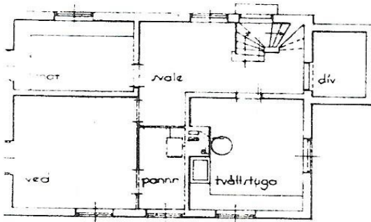
källarplan
