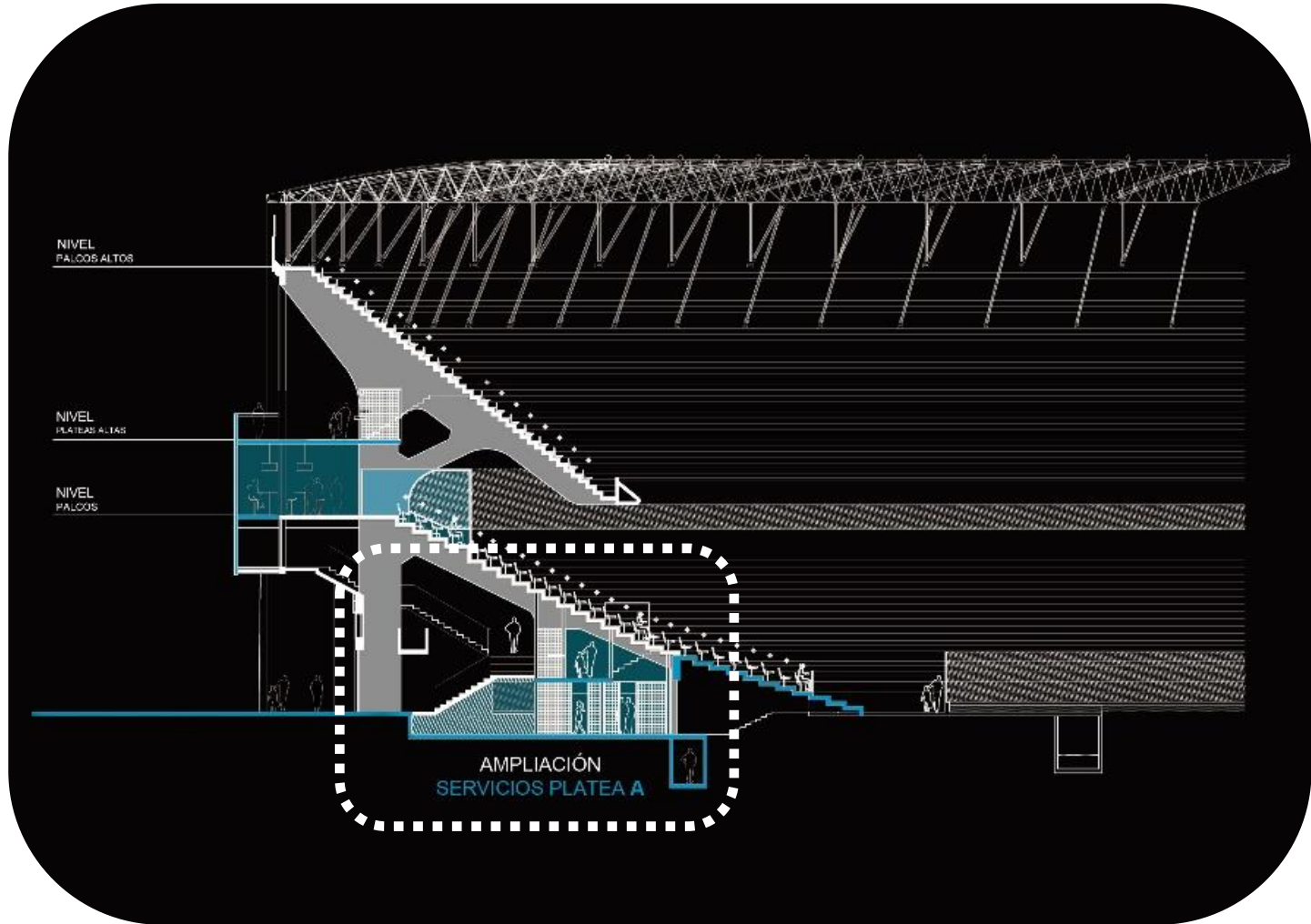
AMPLIACION SERVICIOS SANITARIOS Y GASTRONOMICOS PLATEAS BAJAS.
