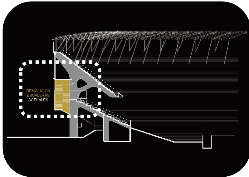
DEMOLICION DE ESCALERAS ACTUALES.
