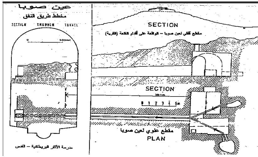
عين صوبيا - رسم د. تسفي رون - الدائرة الجغرافية - جامعة تل أبيب مخطط النبعة ومجمع الماء - مخطط طريق النفق - ومقطع علوي لعين صوبيا
