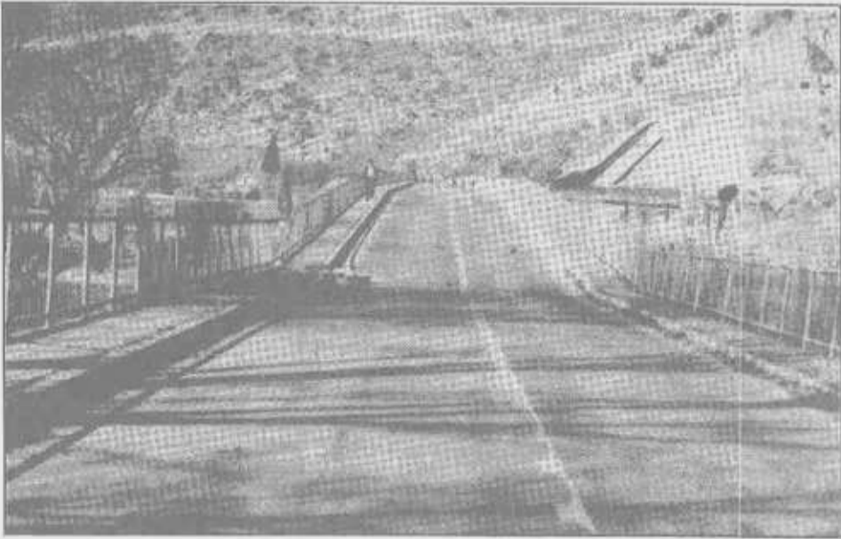
Glavna konstrukcija izdržala — jedan stub poklekao: most u Žitomisliću nakon miniranja
