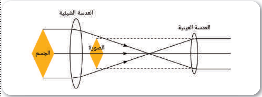
الشكل 5-3 العدسة العينية والشبيئية في التلسكوب.
