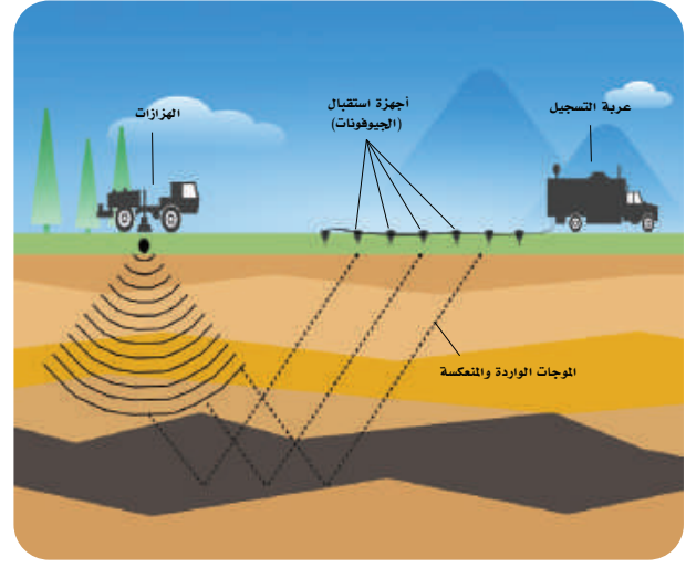
الشكل 7-5 المسح الزلزالي.
