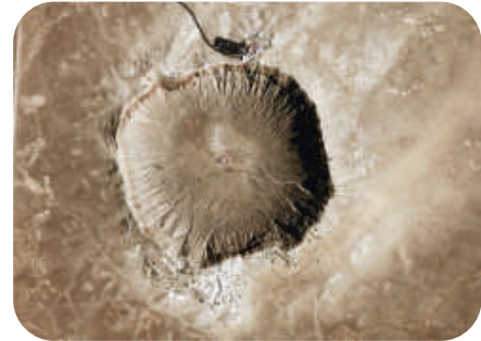
الشكل 14-1 صورة لفوهة ناتجة عن ارتطام نيزك في ولاية أريزونا، الولايات المتحدة الأمريكية.
