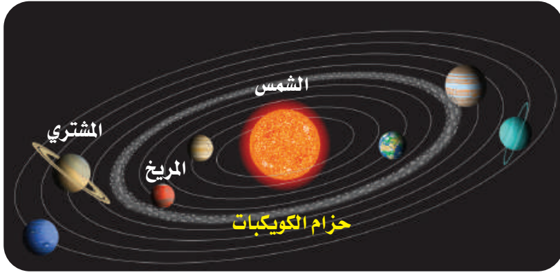
الشكل 11-1 موقع حزام الكويكبات.
