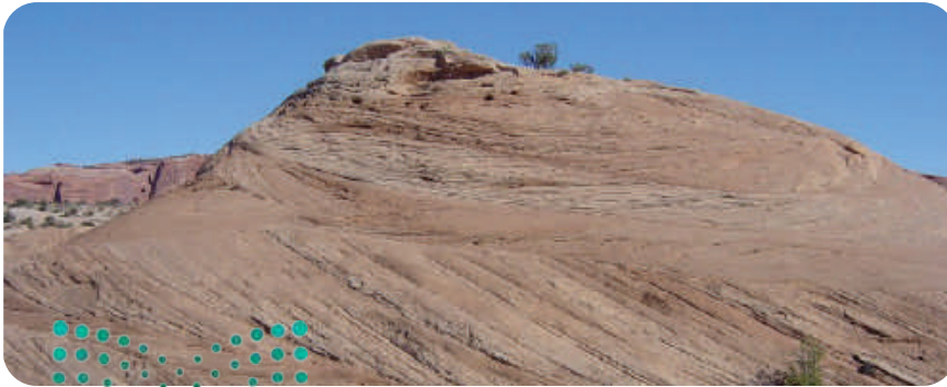
الشكل 22-4 تطبق متقاطع كبير الحجم في كثبان قديمة تشكلت بالرياح.
