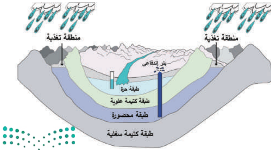
الشكل 16-6 الطبقة المحصورة.
