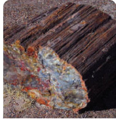
الشكل 7-4 جذع شجرة تم إحلال السيليكا بدل المادة العضوية.
