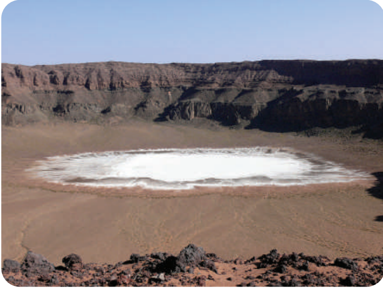
الشكل 9-6 تمثل فوهة الهتيمية في منطقة حائل إحدى الفوهات البركانية المنهارية، ويتراكم على سطحها كميات من الملح نتيجة تبخر المياه التي تتجمع فيها.
