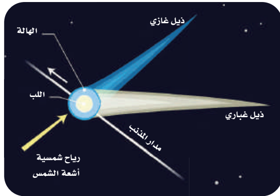
الشكل 1-20 تركيب المذنبات.
