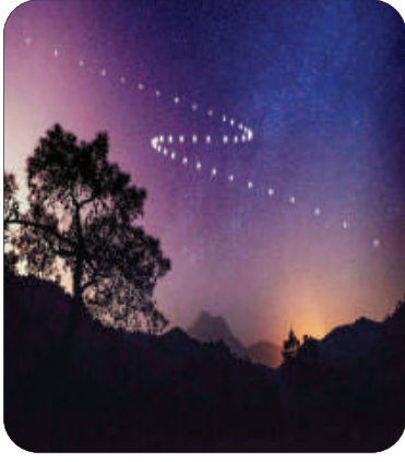
الشكل 7-1 حركة تراجمية مدارية ظاهرية لكوكب المريخ.
