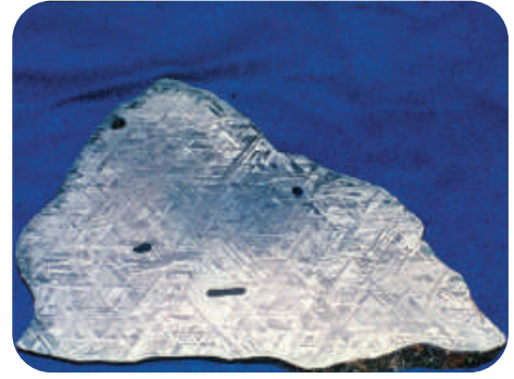
الشكل 1-16 نيزك حديدي. المصدر: وكالة ناسا.
