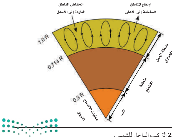
الشكل 2-3 التركيب الداخلي للشمس.
