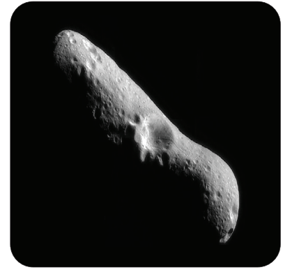
الشكل 12-1 صورة لكويكب إيروس.
