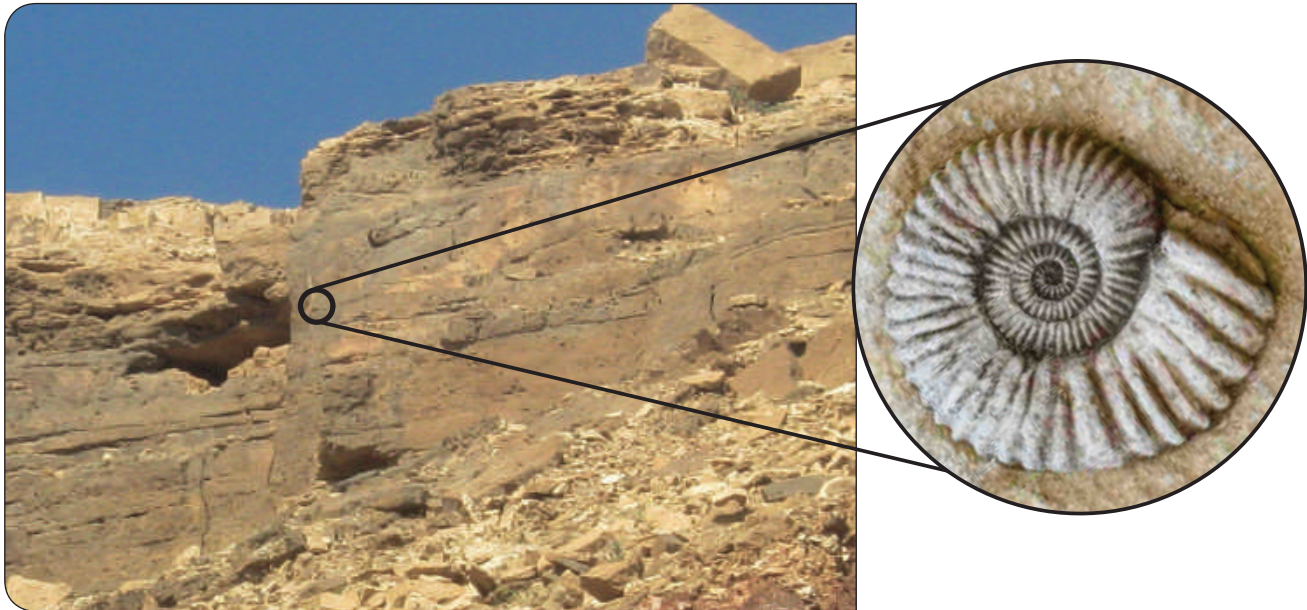
الشكل 28-4 يمكن لصخر الحجر الجيري أن يحوي أنواعاً كثيرة ومختلفة من الأحافير. ويستطيع الجيولوجيون أن يفسروا أين ومتى تشكل الحجر الجيري من دراسة الأحافير الموجودة فيه.
