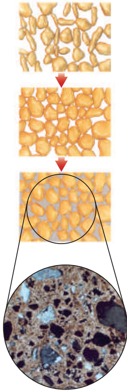
الشكل 20-4 تترسب المعادن من المياه في أثناء تدفقها عبر مسامات الرسوبيات. تشكّل هذه المعادن مادة لاحمة تعمل على ربط الرسوبيات بعضها مع بعض.
